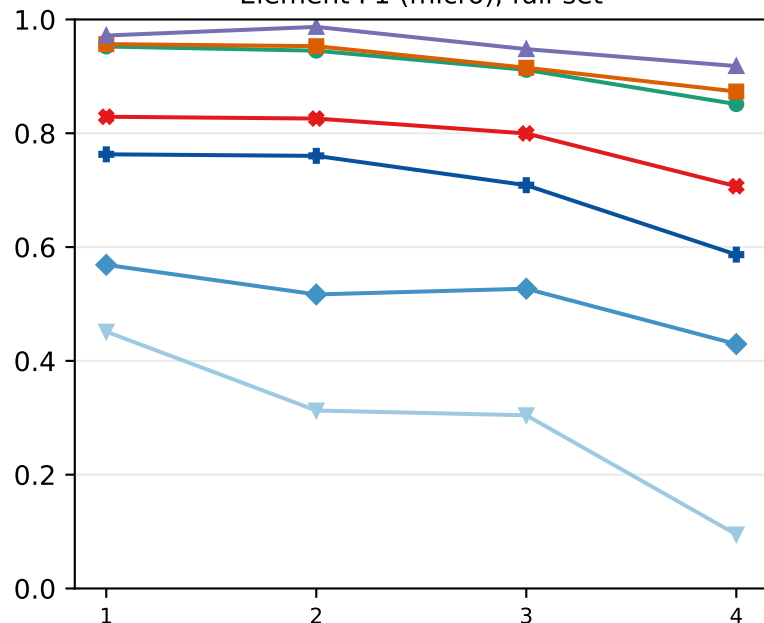
Element F1 (micro), full-set
