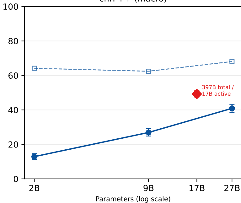
chrF++ (macro)
