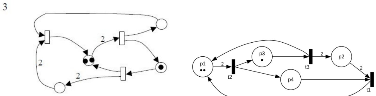
Рисунок 1: Ліворуч — вирізка оригінального рисунка мережі варіанта 3 (с. 6 умови); праворуч — та сама мережа, перемальована з явними іменами позицій і переходів; фішки \mu_0 показані крапками.
