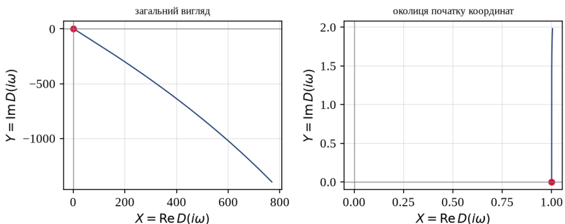
Рисунок 5: Годограф Михайлова для D(p) = p^{10} + 7p^8 + 11p^7 + 5p + 1 : ліворуч — хід кривої на \omega \in [0; 2] , праворуч — та сама крива в околиці початку координат, \omega \in [0; 0.4]
