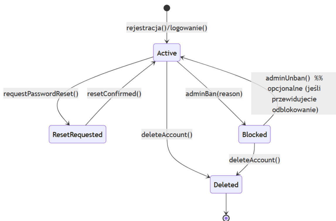
Rysunek 1: Diagram stanów: User.
