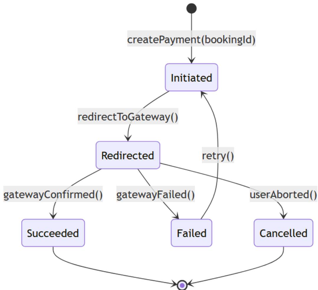
Rysunek 4: Diagram stanów: Payment.
