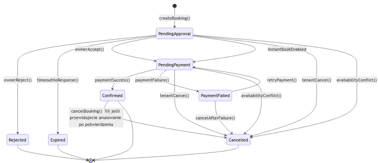
Rysunek 3: Diagram stanów: Booking.
