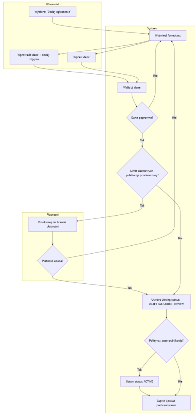
Rysunek 6: Diagram aktywności: Wystawienie ogłoszenia (Create Listing).
