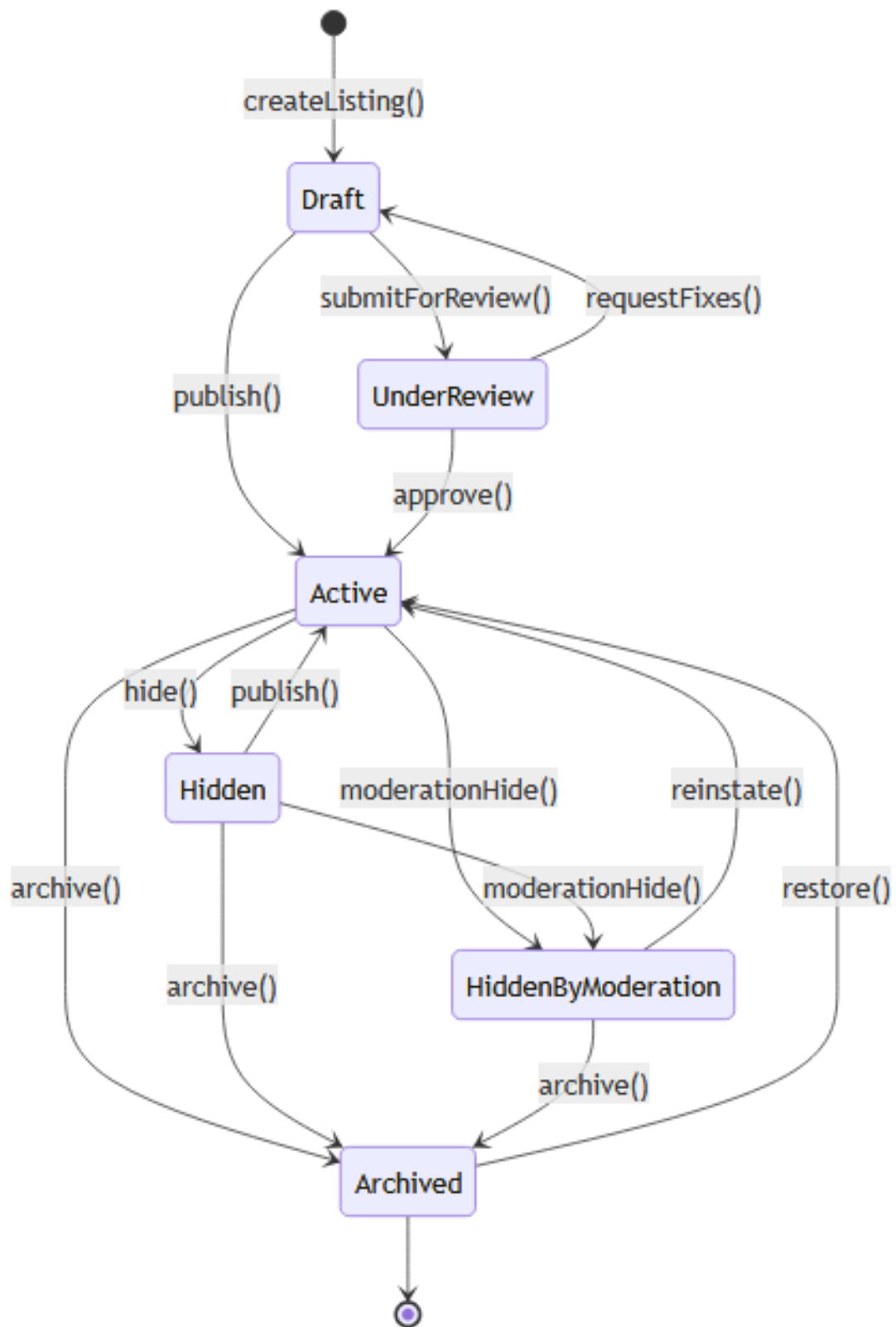
Rysunek 2: Diagram stanów: Listing.
