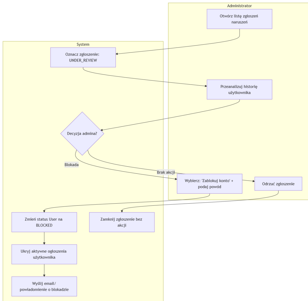
Rysunek 9: Diagram aktywności: Blokada użytkownika (Ban User).
