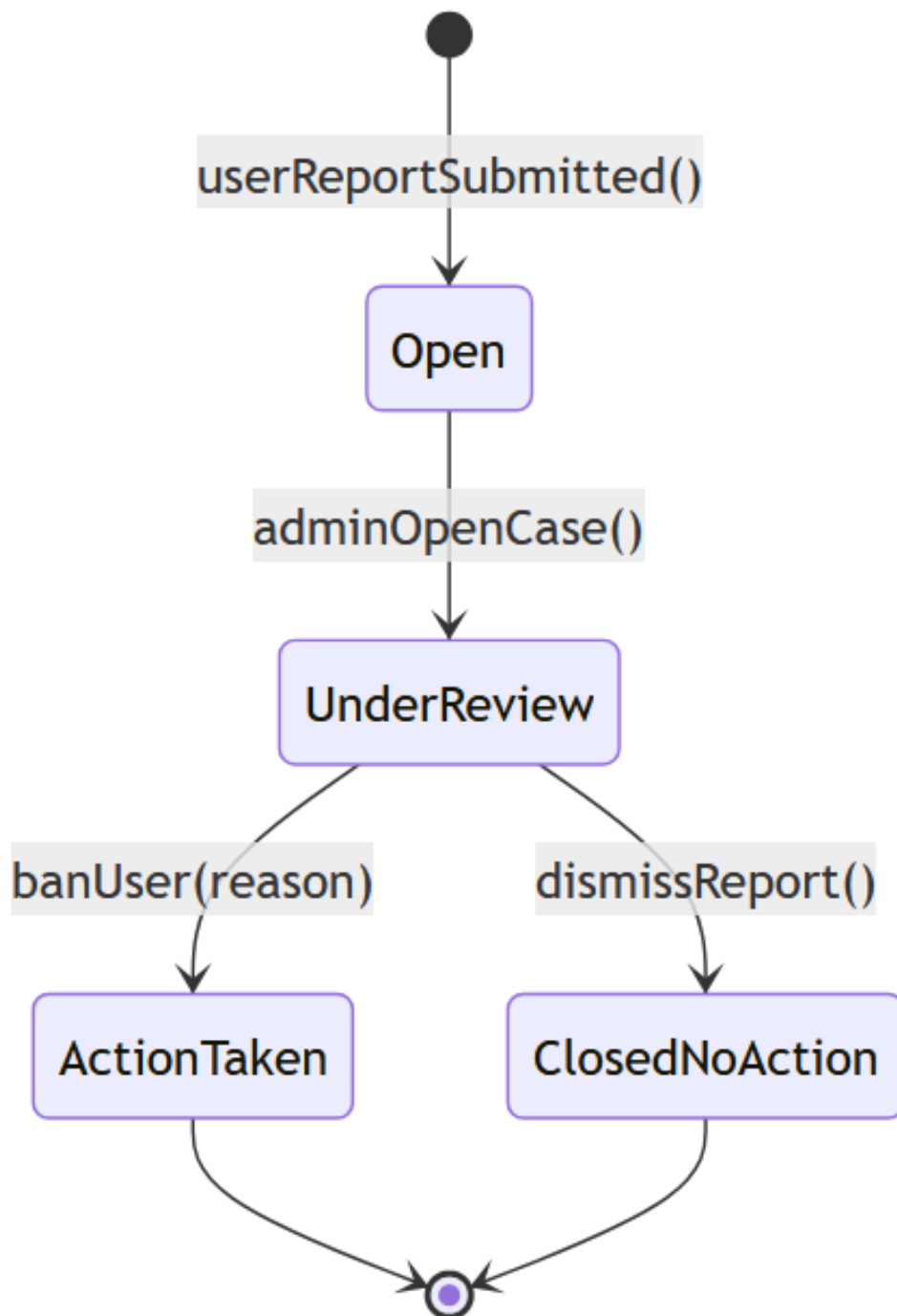
Rysunek 5: Diagram stanów: ViolationReport.
