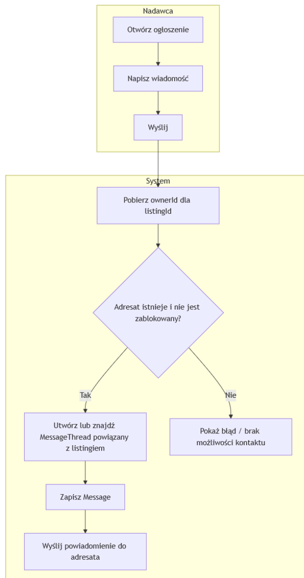
Rysunek 8: Diagram aktywności: Wysyłanie wiadomości w kontekście ogłoszenia.
