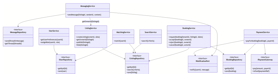
Rysunek 6: Diagram klas - serwisy, repozytoria i porty integracyjne (płatności, powiadomienia)
