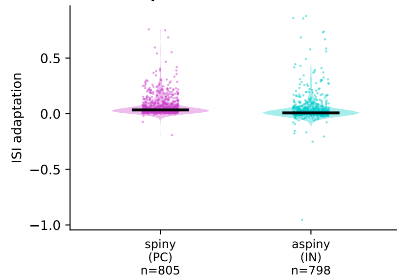
L. ISI adaptation
