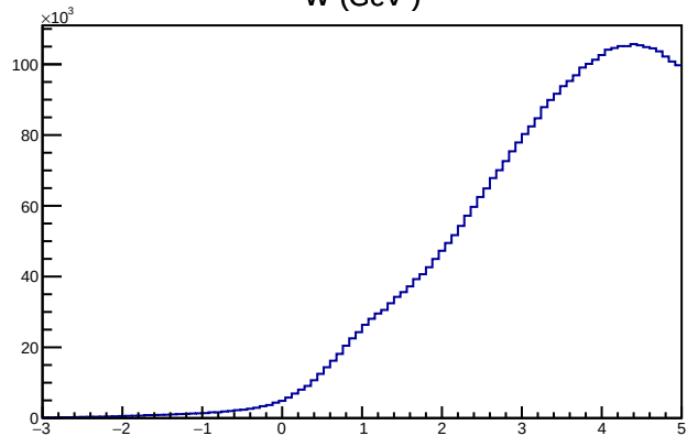
W^2(\text{GeV}^2)
