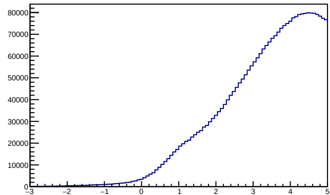
W^2(\text{GeV}^2)
