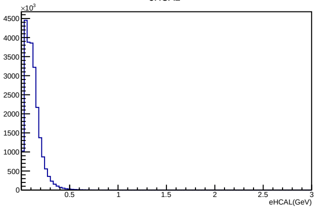
eHCAL
