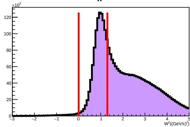
W^2
