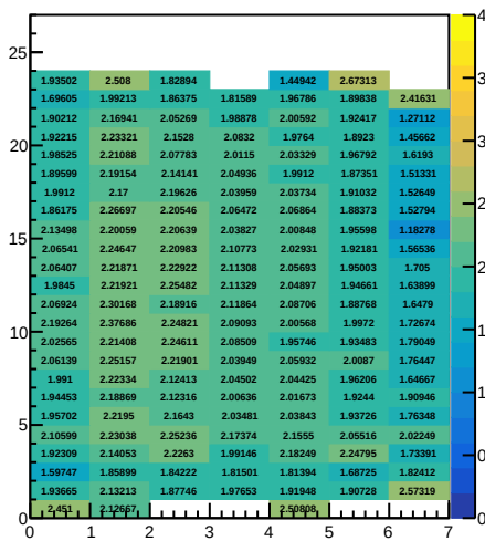
SH energy per SH block
