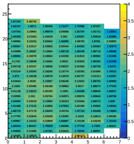
SH energy per SH block
