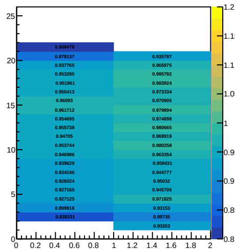
E/p per PS block
