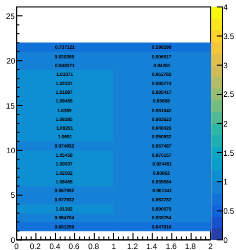
PS energy per PS block
