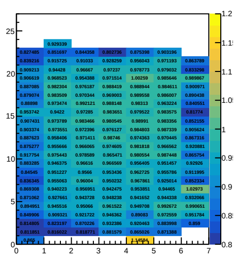
E/p per SH block
