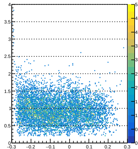
PS energy vs Track y (proj. at PS)
