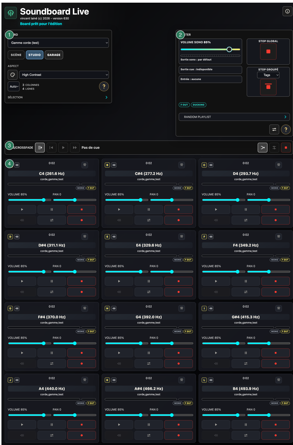
Mode Studio (skin high contrast) — 1 Board et versions · 2 Master (commandes globales) · 3 Bloc Cues/Crossfade · 4 Pads
