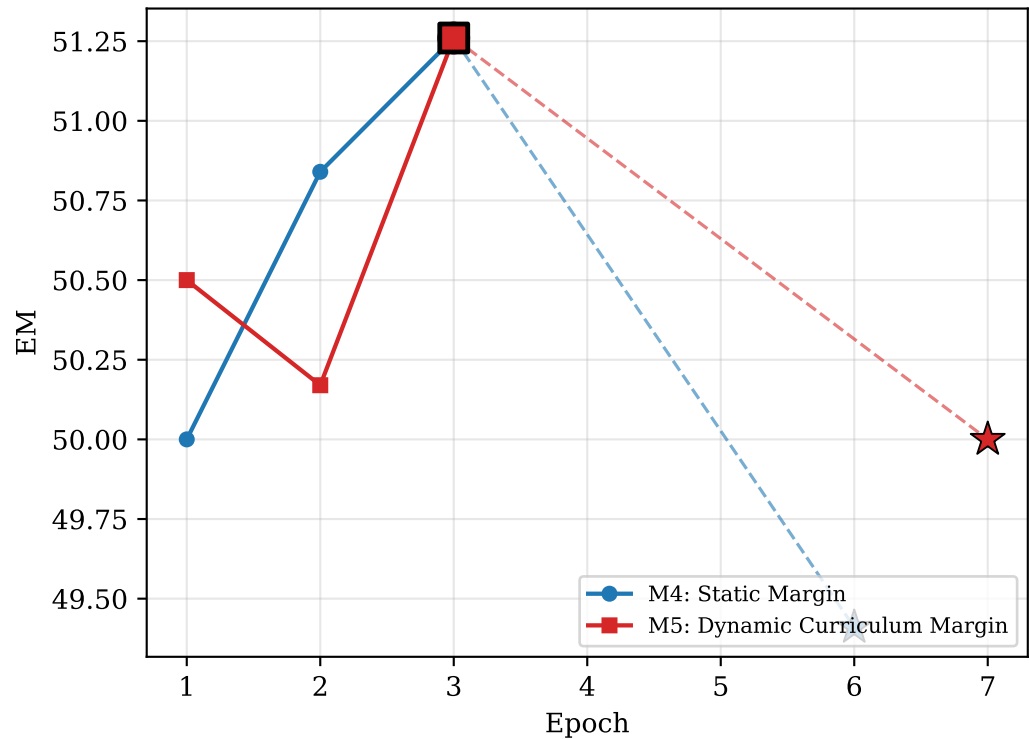
XQuAD-VI: Validation EM vs. Epoch
