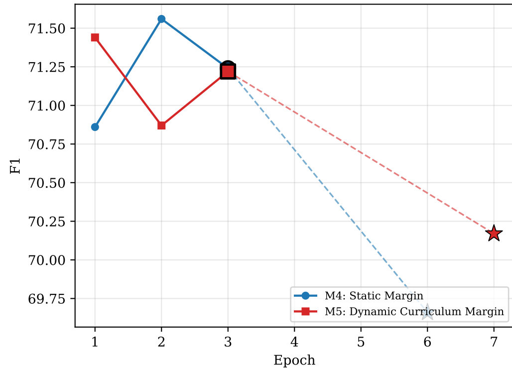
XQuAD-VI: Validation F1 vs. Epoch
