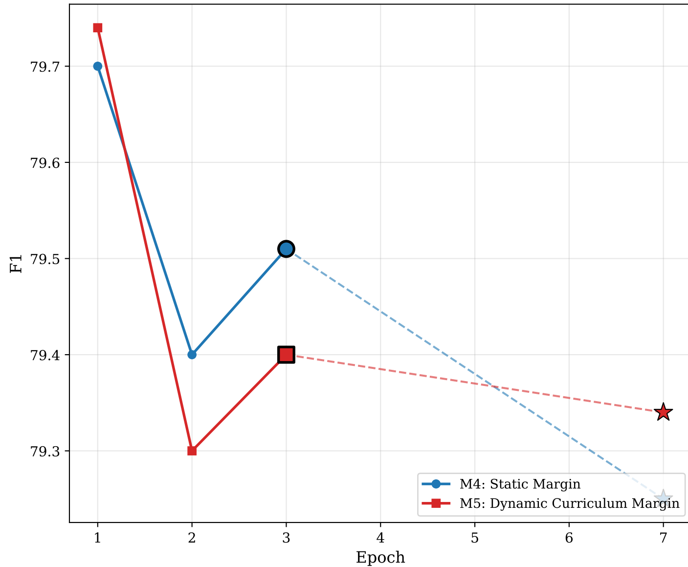
MLQA-en: Validation F1 vs. Epoch
