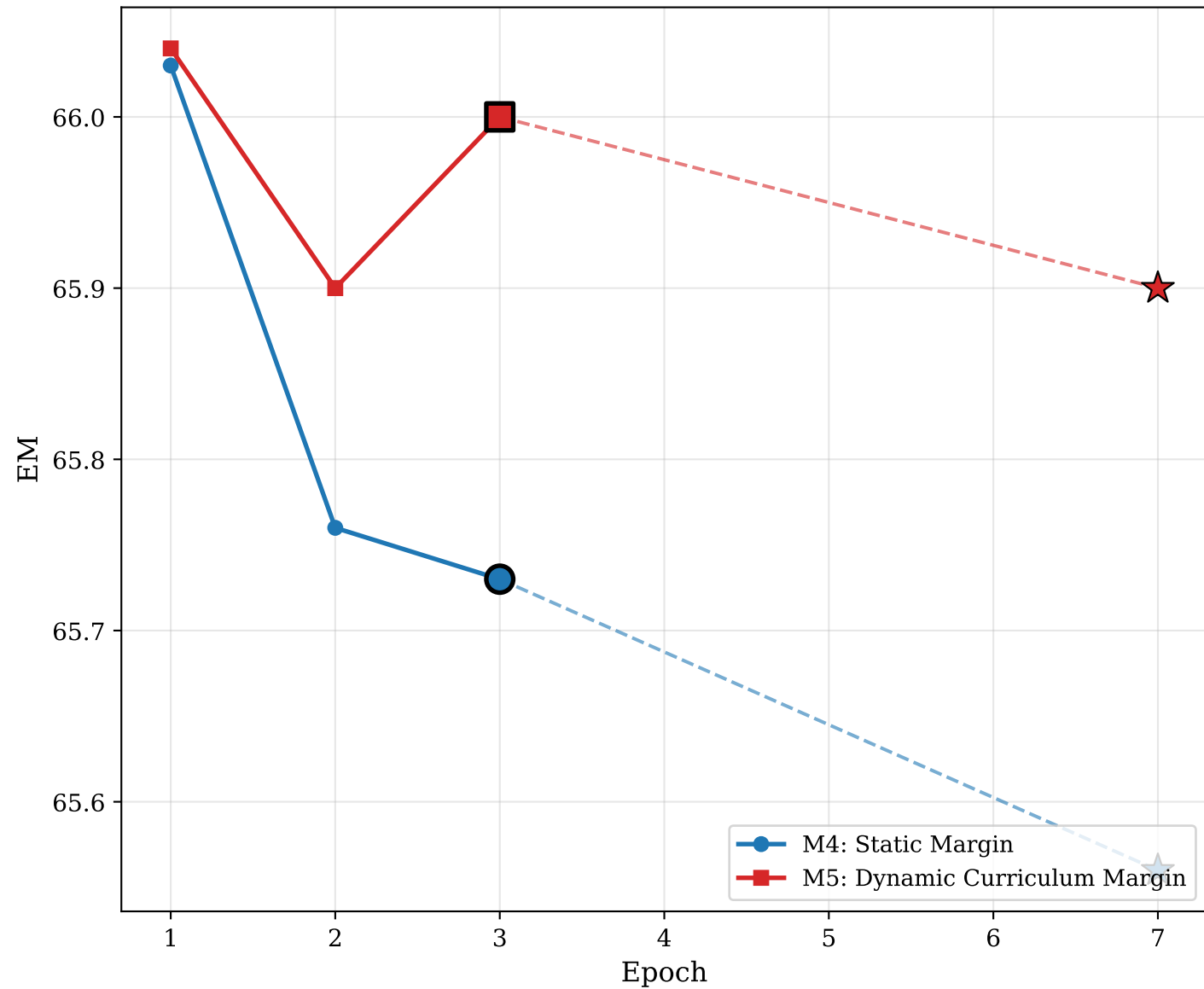
MLQA-en: Validation EM vs. Epoch
