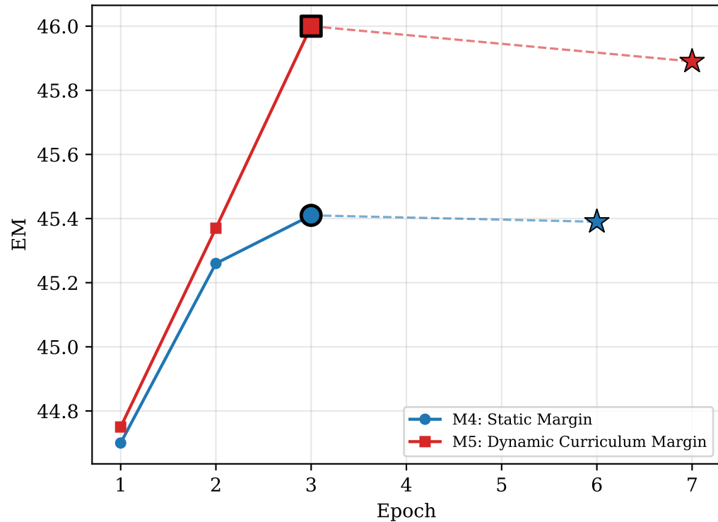
MLQA-vi: Validation EM vs. Epoch
