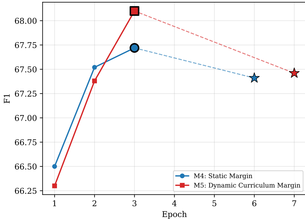
MLQA-vi: Validation F1 vs. Epoch
