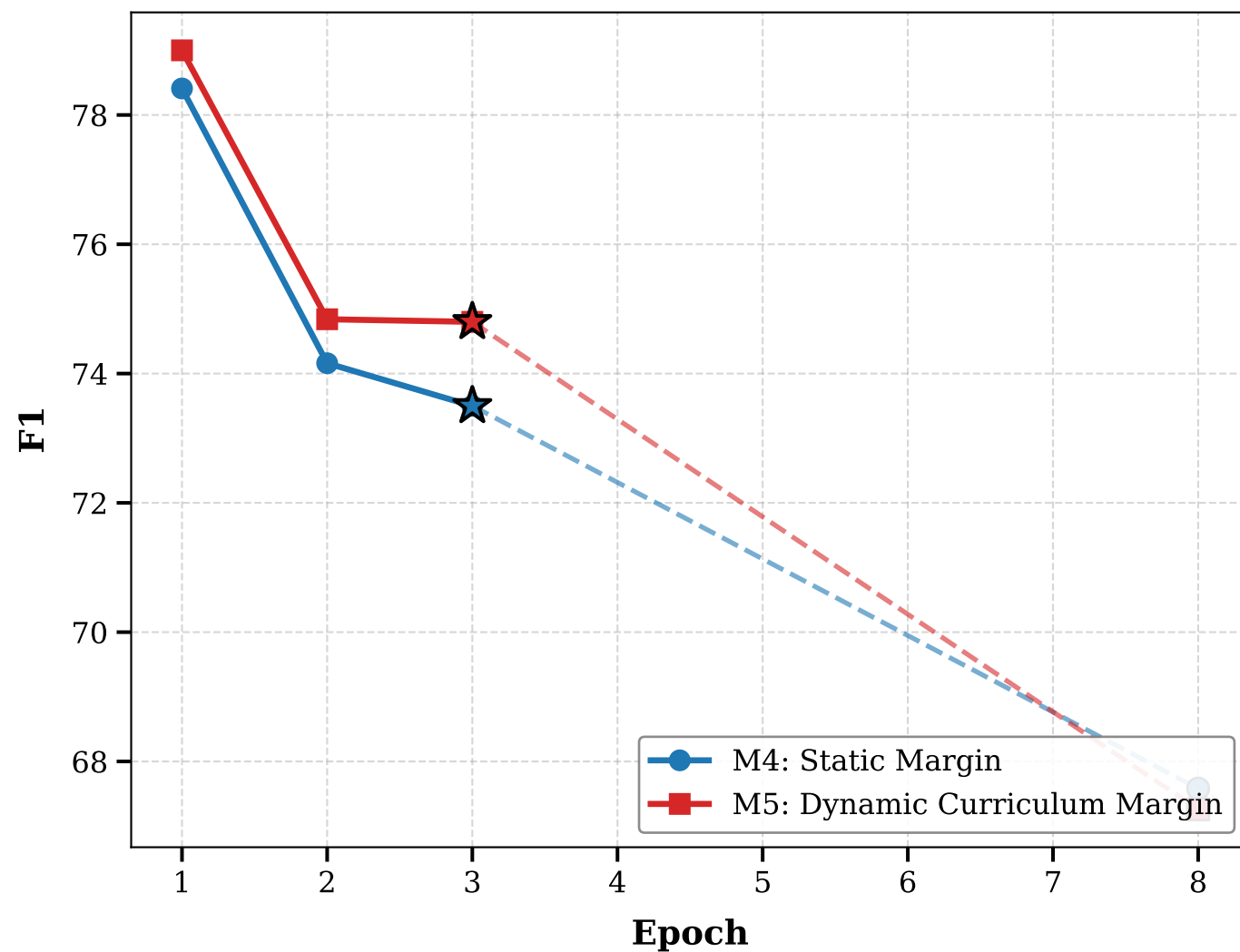
MLQA-en: Validation F1 vs. Epoch
