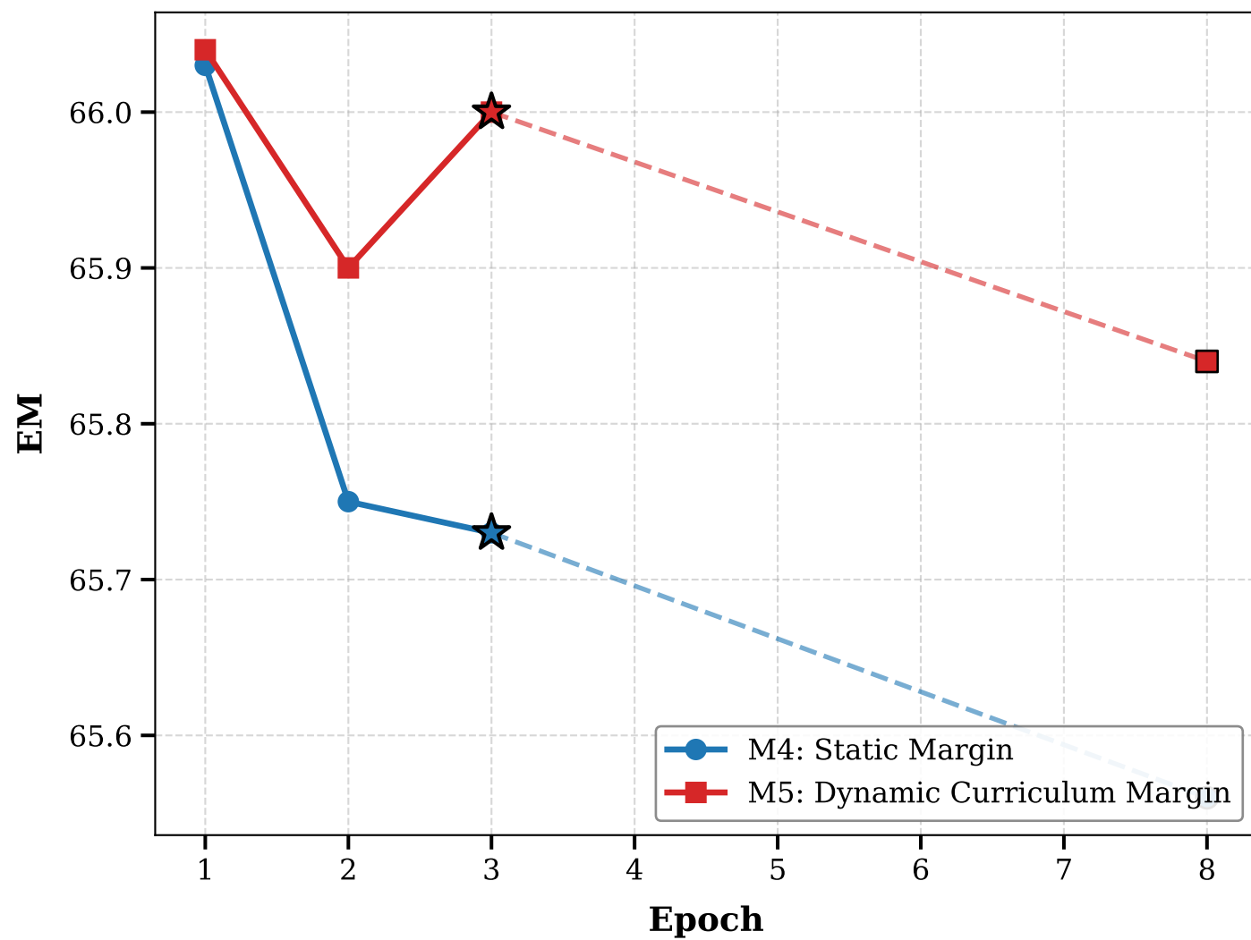
MLQA-en: Validation EM vs. Epoch
