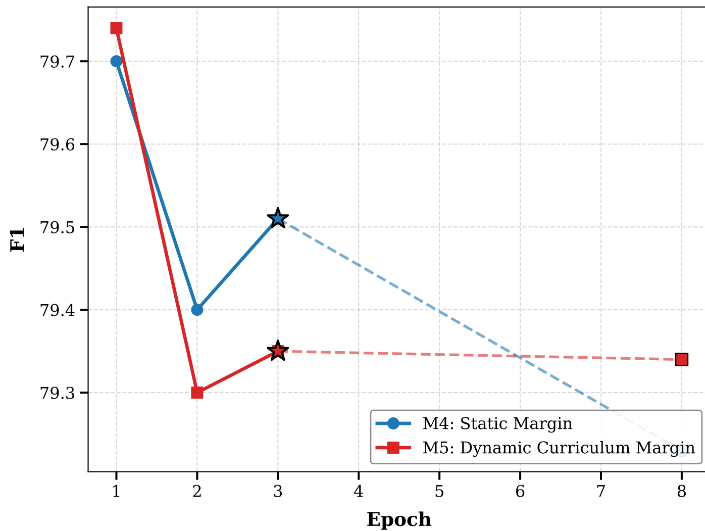
MLQA-en: Validation F1 vs. Epoch
