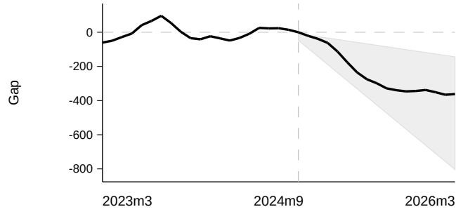
(c) Bolsa Família: Gap e IC 90%
