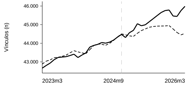
(b) Estoque formal: Observado e sintético
