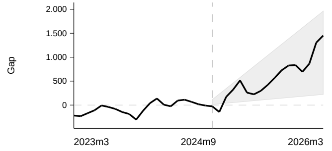
(d) Estoque formal: Gap e IC 90%
