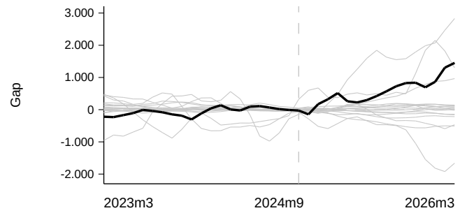
(f) Estoque formal: Placebos
