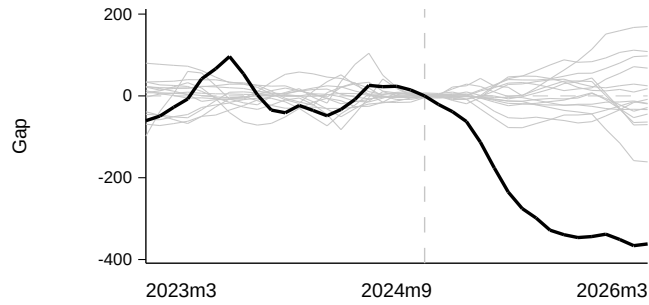
(e) Bolsa Família: Placebos
