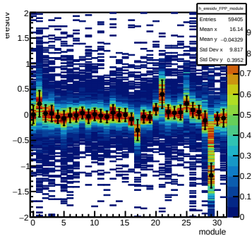
eresidv FPP
