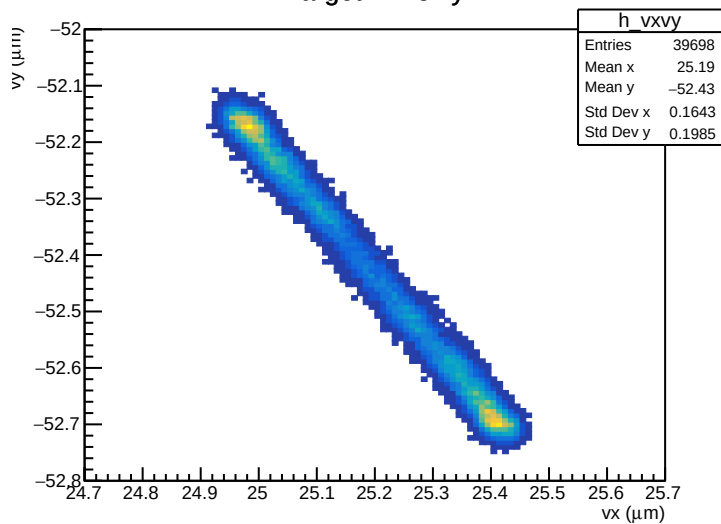
Target vx vs vy
