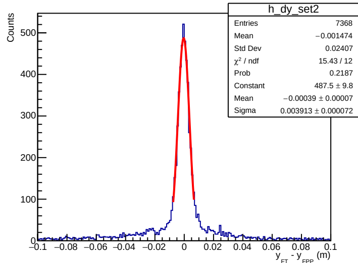
Track \Delta Y
