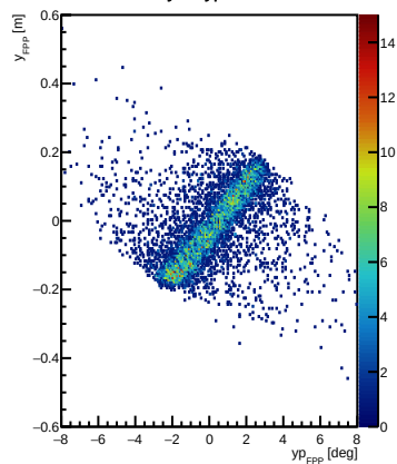
y vs y_P FPP
