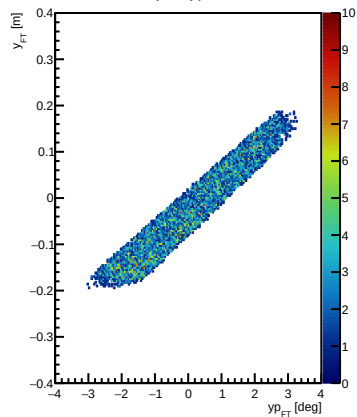
y vs y_P FT
