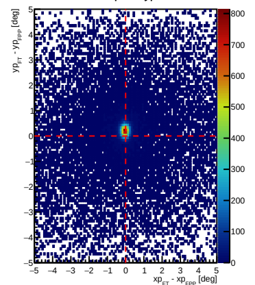
dxp vs dyp
