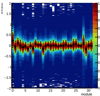
eresidu FPP
