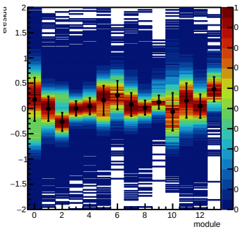
eresidu FT
