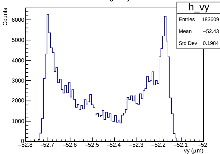
Target vy
