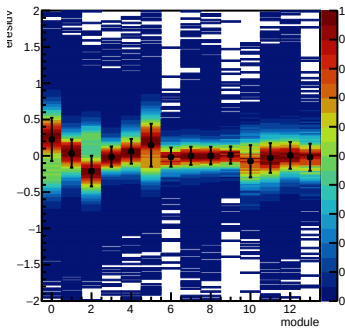
eresidv FT
