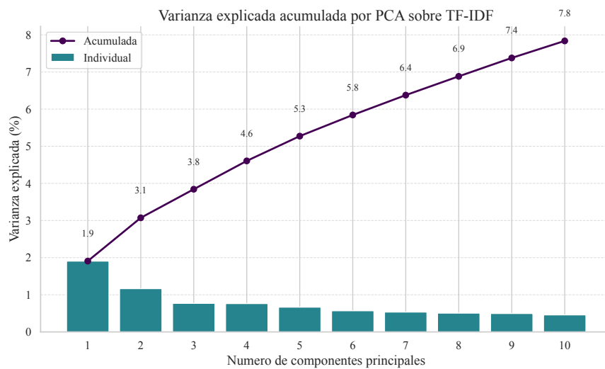
Figura 3: Varianza explicada individual y acumulada en función de la cantidad de componentes principales. Con diez componentes apenas se alcanza un 7,8% de varianza explicada.
