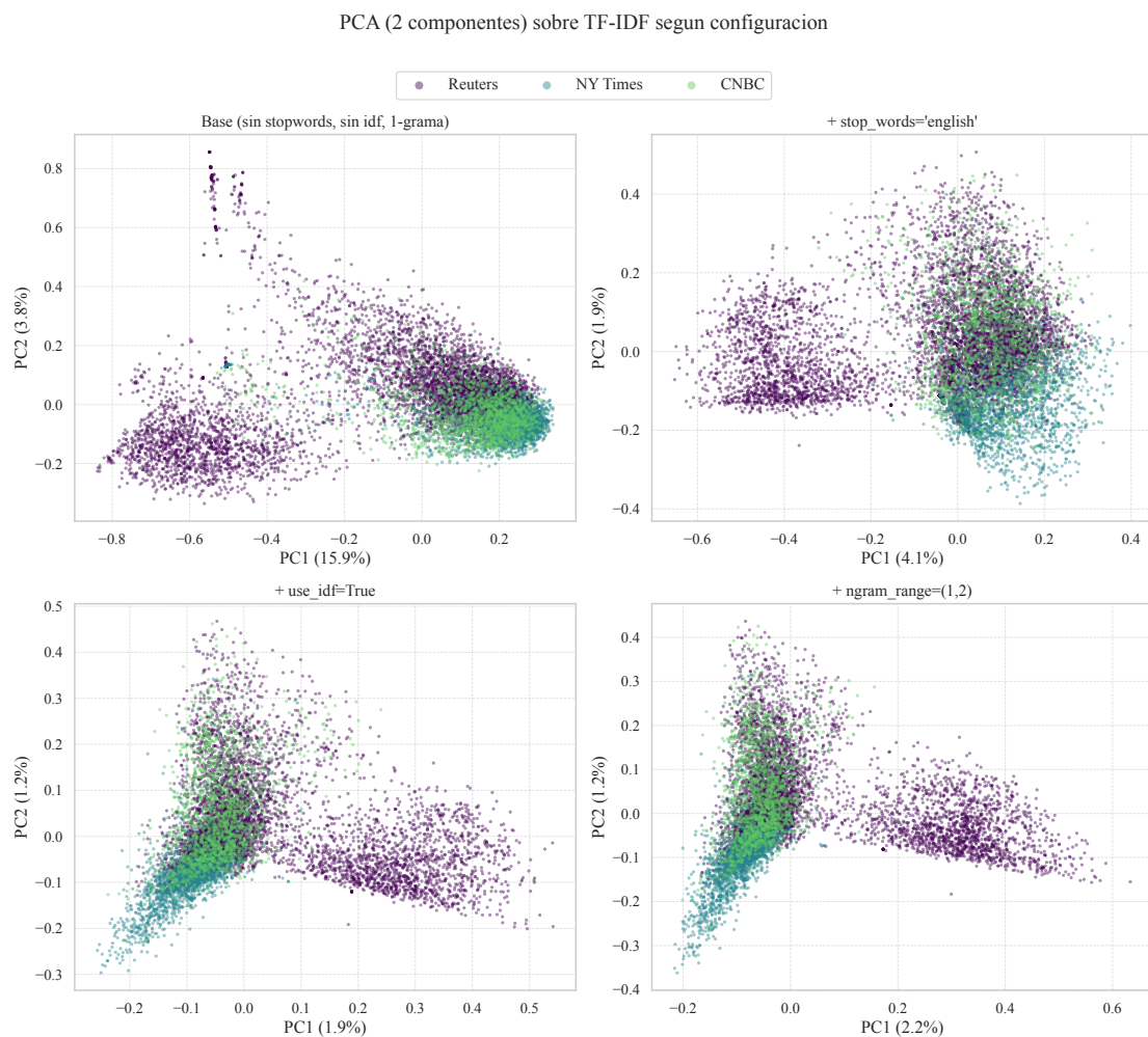
Figura 2: Proyección de los artículos de entrenamiento sobre las dos primeras componentes principales del TF-IDF, para distintas configuraciones del vectorizador. Entre paréntesis se indica la varianza explicada por las dos componentes en cada caso.
