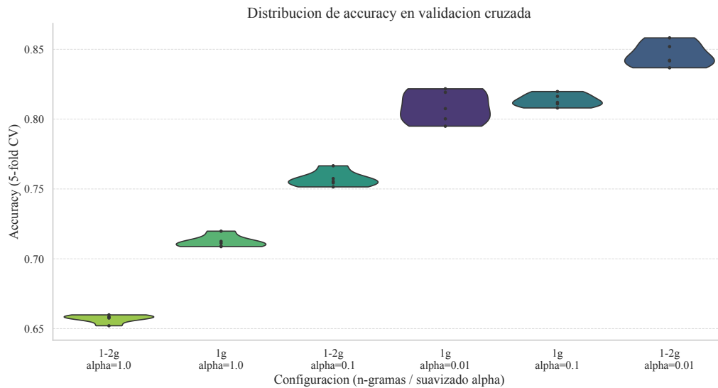
Figura 5: Distribución de la accuracy en los cinco folds de validación cruzada para cada configuración evaluada en la búsqueda de hiperparámetros.
