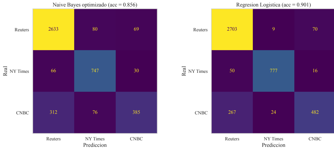
Figura 6: Matrices de confusión sobre el conjunto de test del Naive Bayes optimizado (izquierda) y de la Regresión Logística (derecha). Esta última reduce de forma apreciable las confusiones de CNBC .
