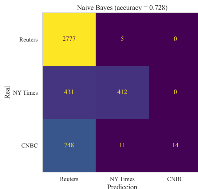
Figura 4: Matriz de confusión del modelo Naive Bayes con parámetros por defecto. Prácticamente todos los artículos de CNBC son asignados a Reuters.
