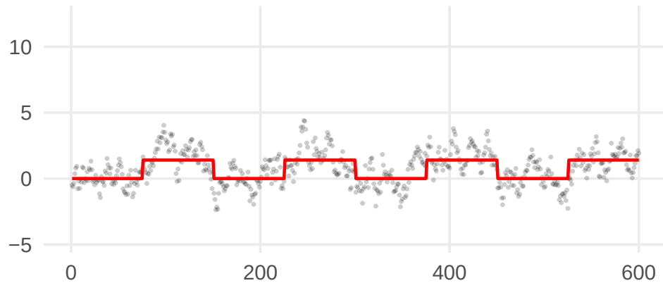
updown
