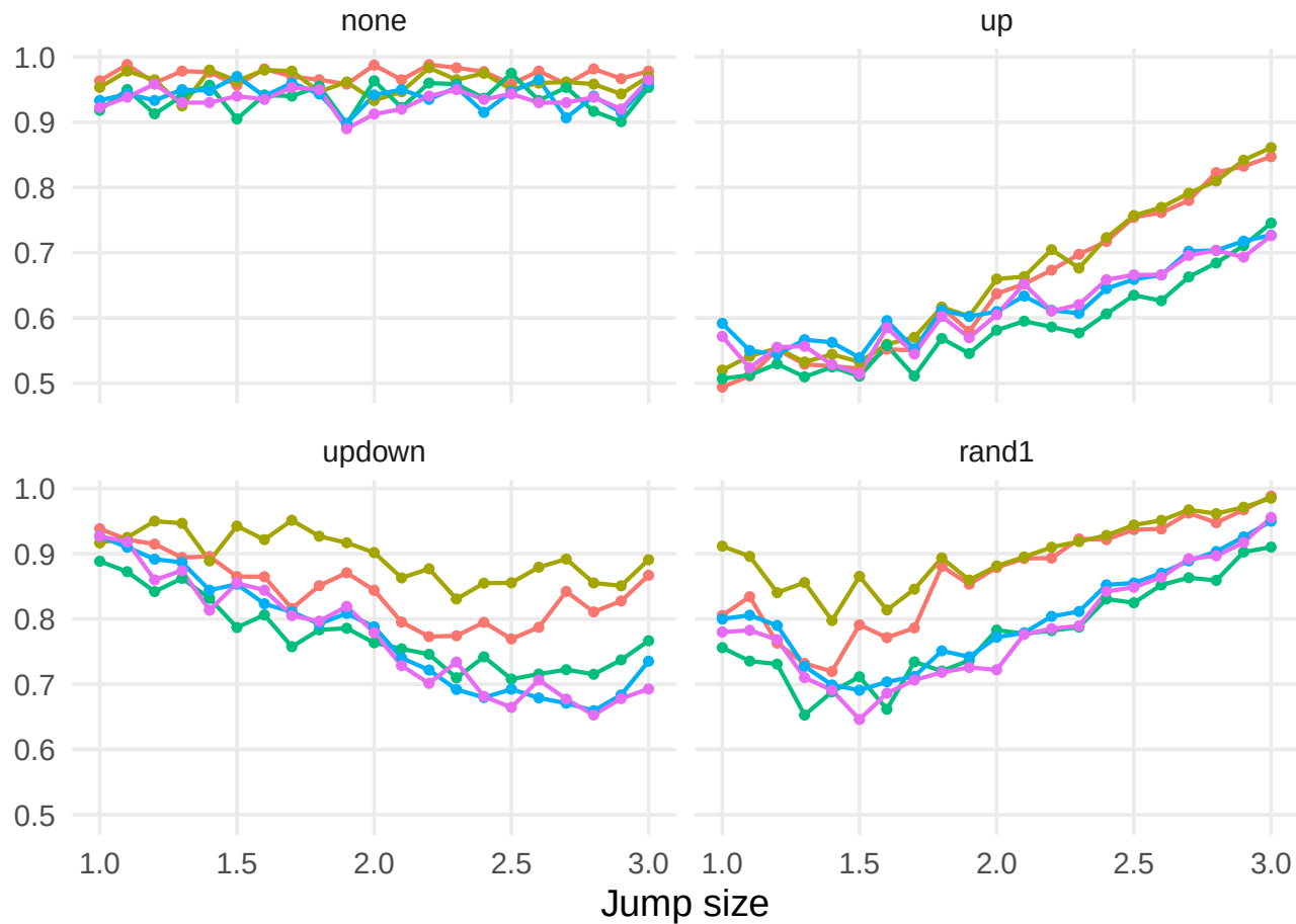
Precision
