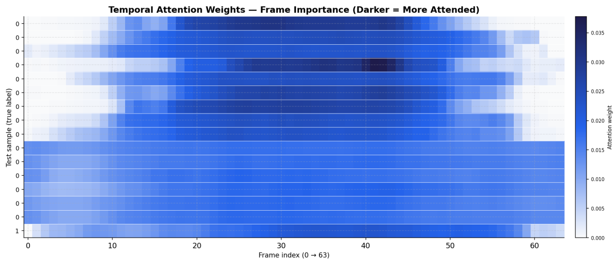
Hình 5.5: Biểu đồ trọng số Temporal Attention theo từng frame
