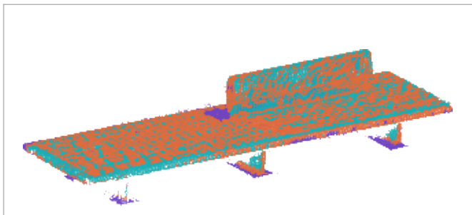
hloc + COLMAP
