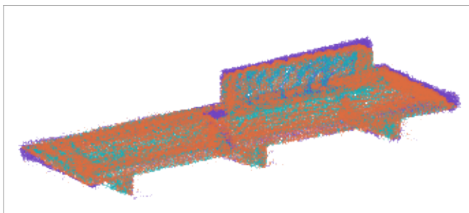
VGGT
