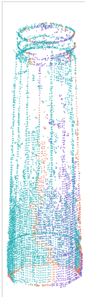
hloc + COLMAP
