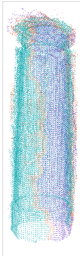
VGGT
