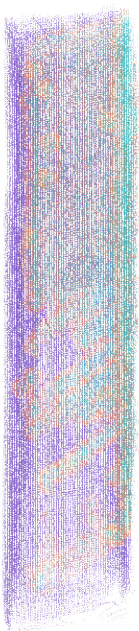
VGGT
