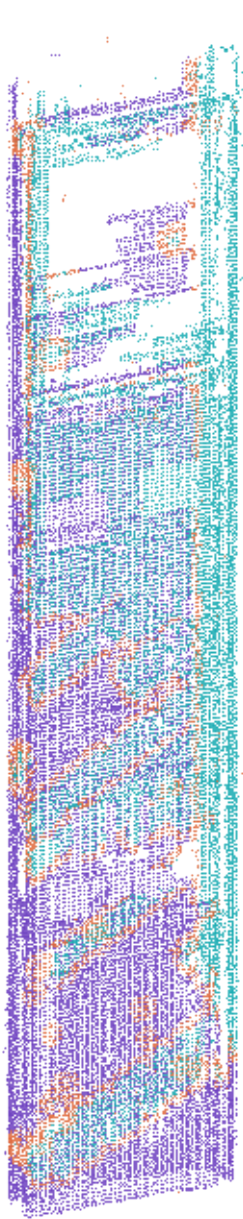
hloc + COLMAP
