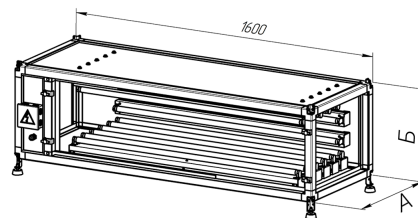
Габаритная схема секции бактерицидной обработки RBW RIK-M
