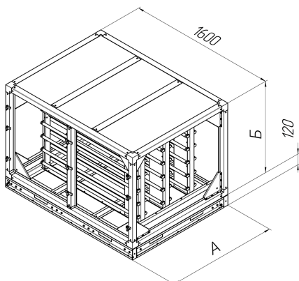
Габаритная схема секции бактерицидной обработки RBW RIK-S
