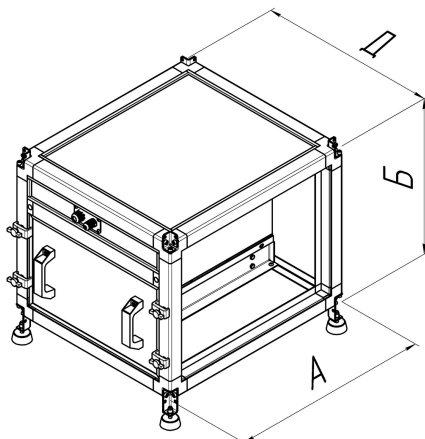
Габаритная схема электрических воздухонагревателей RE RIK-M
