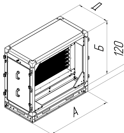
Габаритная схема электрических воздухонагревателей RE RIK-S
