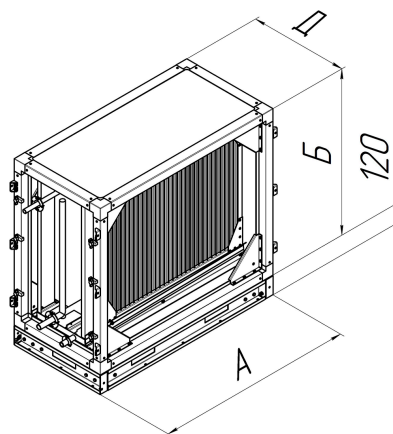
Габаритная схема фреоновых воздухоохладителей RSF RIK-S
