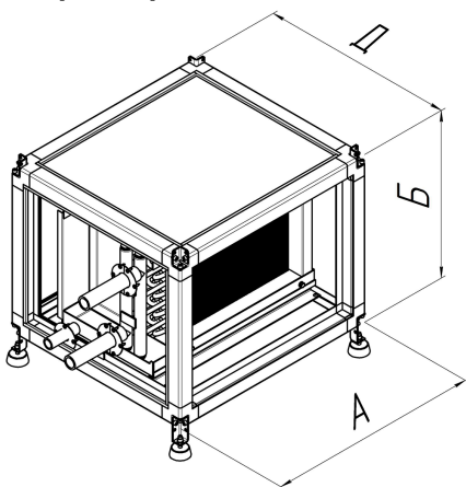
Габаритная схема фреоновых воздухоохладителей RSF RIK-M
