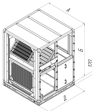
Габаритная схема пластинчатых рекуператоров REC RIK-S
