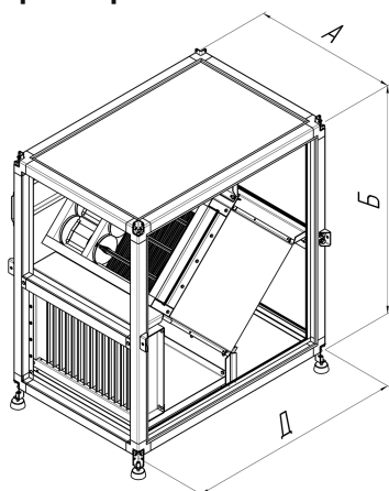
Габаритная схема пластинчатых рекуператоров REC RIK-M
