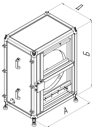
Габаритная схема роторных регенераторов REG RIK-M
