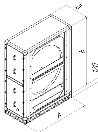
Габаритная схема роторных регенераторов REG RIK-S
