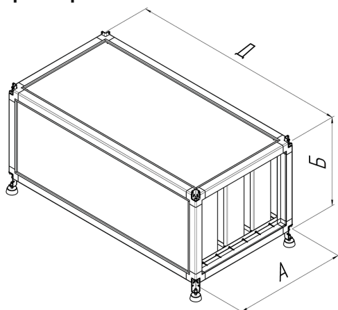
Габаритная схема шумоглушителей RY RIK-M
