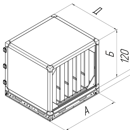
Габаритная схема шумоглушителей RY RIK-S
