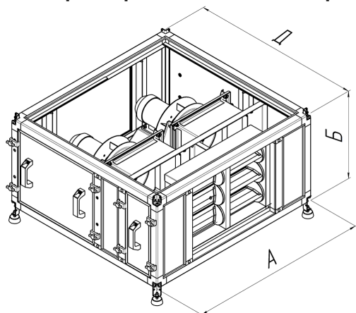
Габаритные схемы вентиляторных секций с резервированием RIK-M
