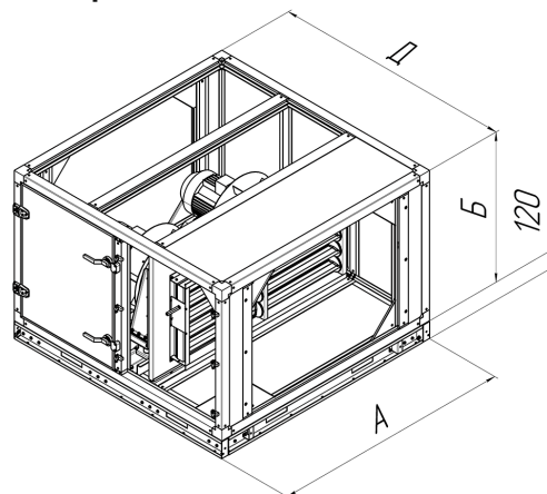
Габаритные схемы вентиляторных секций с резервированием RIK-S
