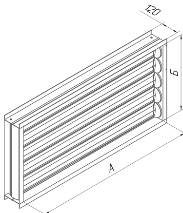
Габаритные размеры секционной регулирующей заслонки RS
