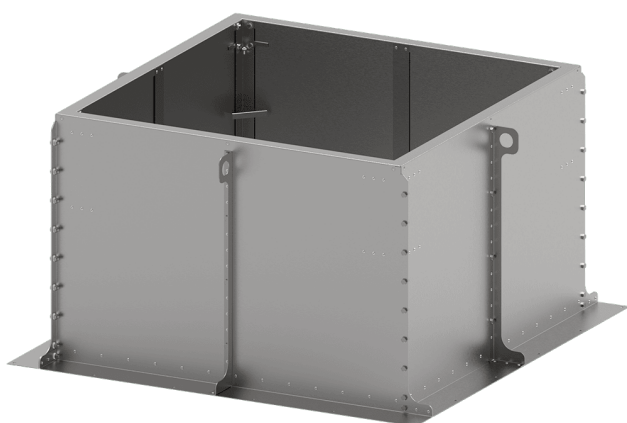
Монтажный стакан (H=1000 мм)
