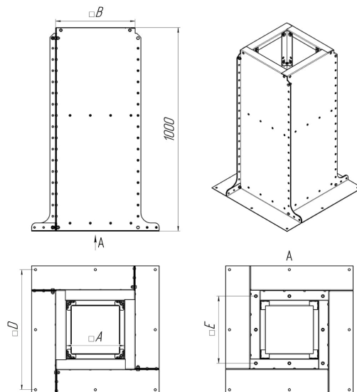
Габаритная схема (H=1000 мм)
