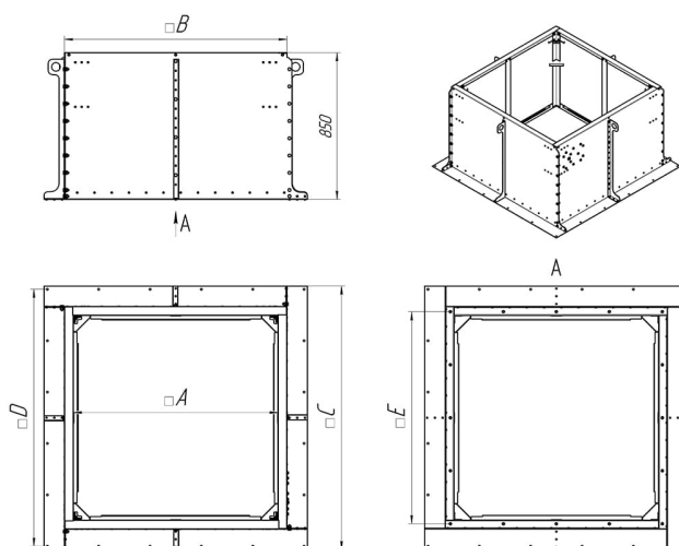
Габаритная схема (H=850 мм)
