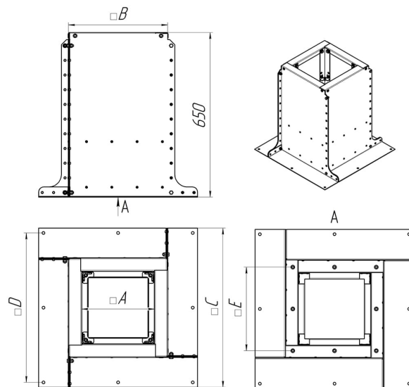
Габаритная схема (H=650 мм)
