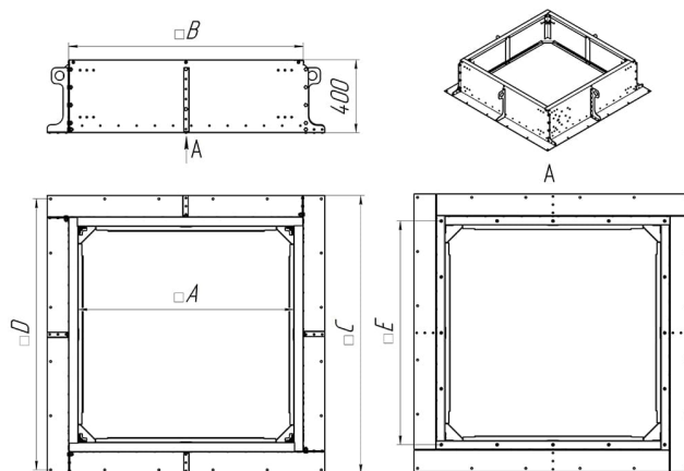
Габаритная схема (H=400 мм)
