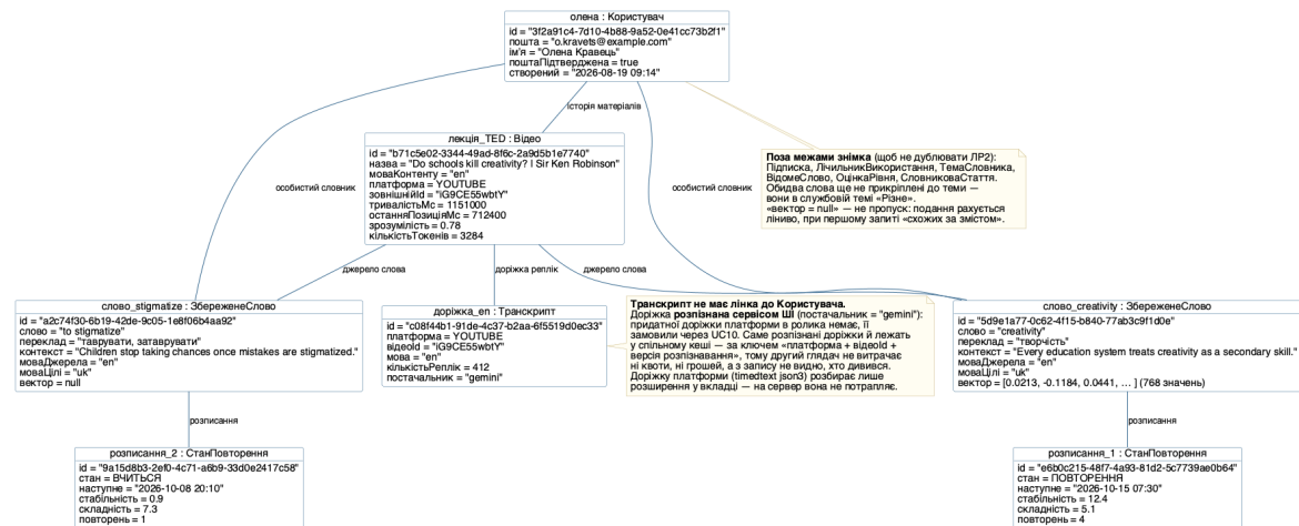
Рисунок 1 — Діаграма об'єктів: знімок стану системи на 8 жовтня 2026 р., 18:42
