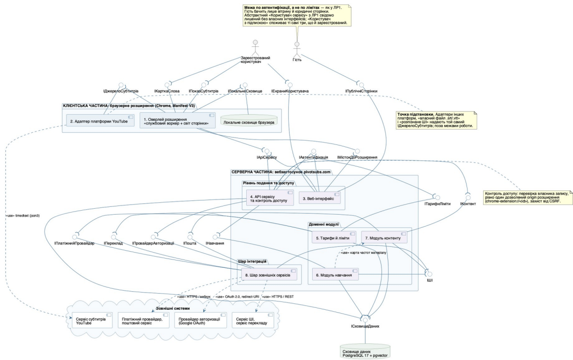
Рисунок 2 — Діаграма компонентів: клієнтська частина (розширення) і серверна частина (вебзастосунок)
