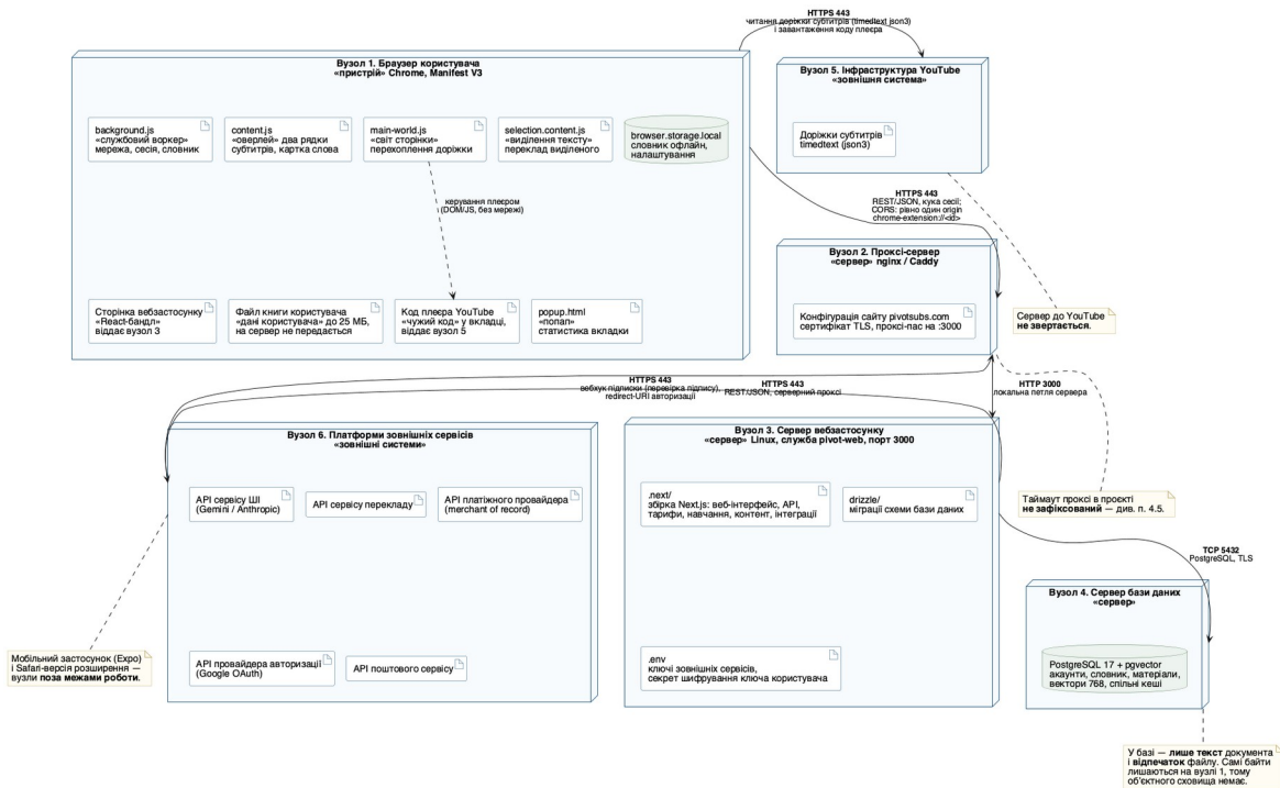
Рисунок 3 — Діаграма розгортання: шість вузлів, артефакти на вузлах і протоколи на зв'язках
