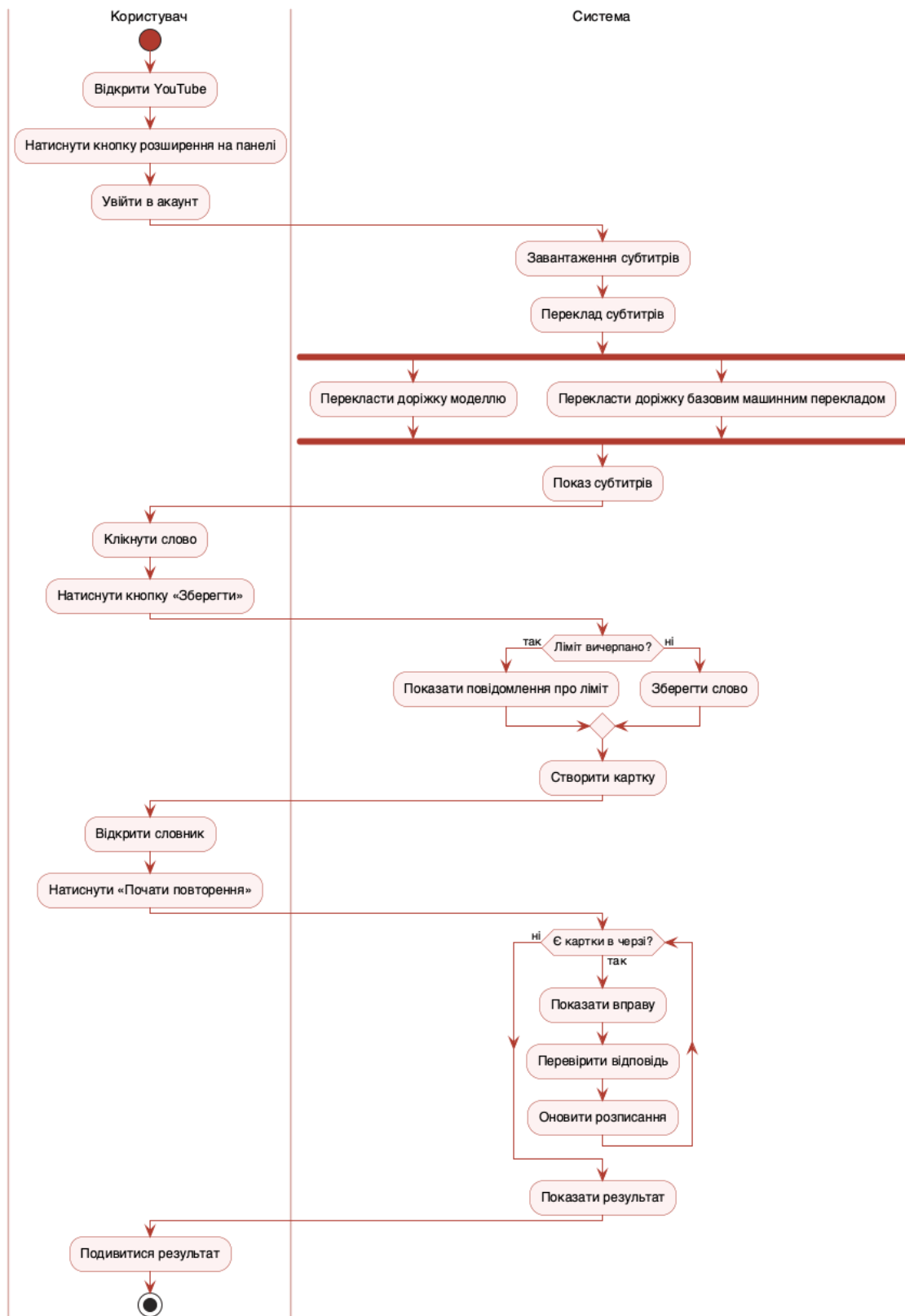
Рисунок 4 — Чернетка діаграми діяльності, згенерована ШІ, з усіма початковими хибками
