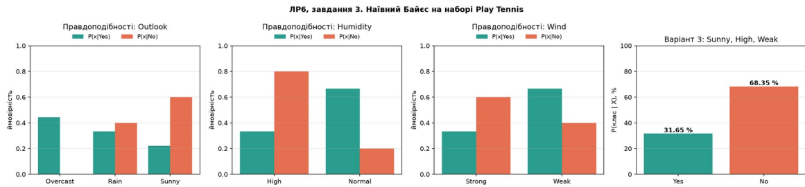
Рисунок 1 — таблиці правдоподібності за атрибутами Outlook, Humidity, Wind і апостеріорні ймовірності для умов варіанта 3
