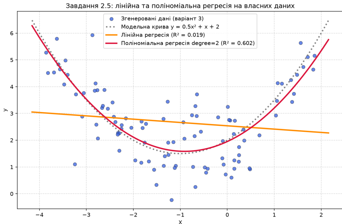
Рисунок 7 — власні дані варіанта 3: лінійна та поліноміальна регресія
