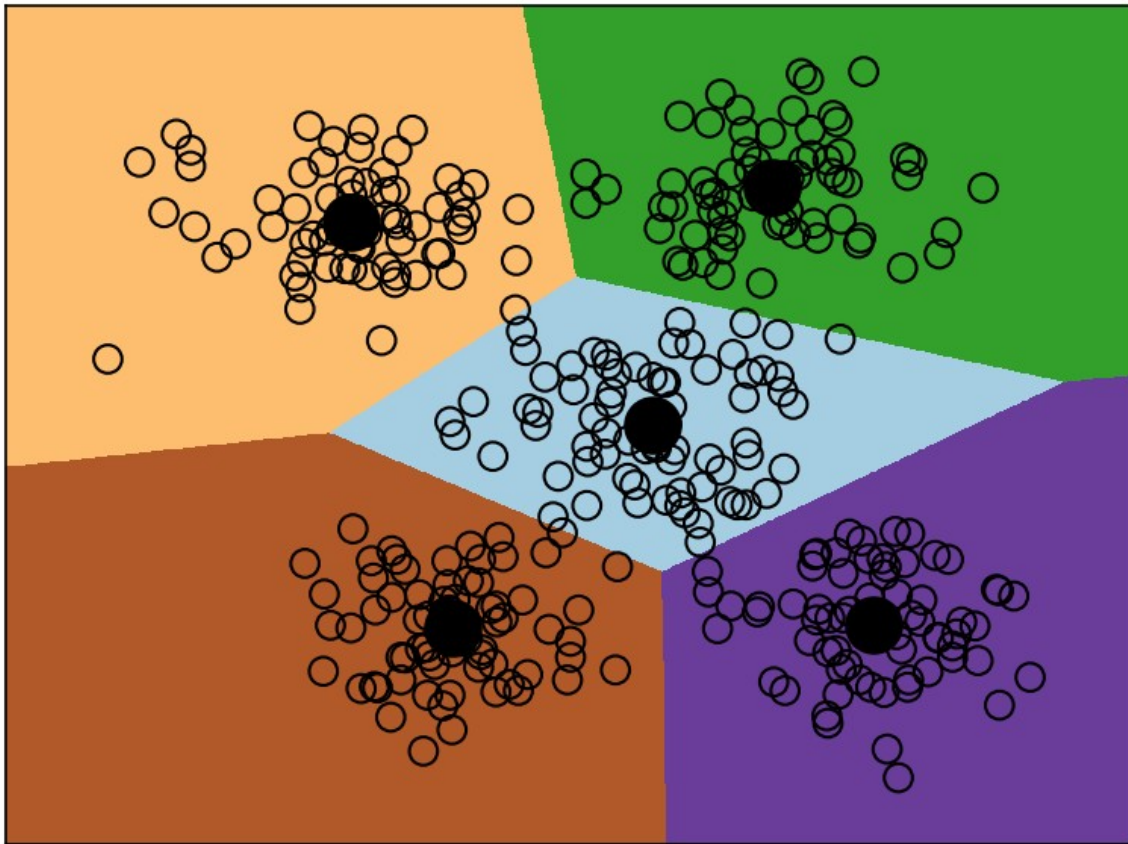
Межі кластерів (k-середніх, k=5)
