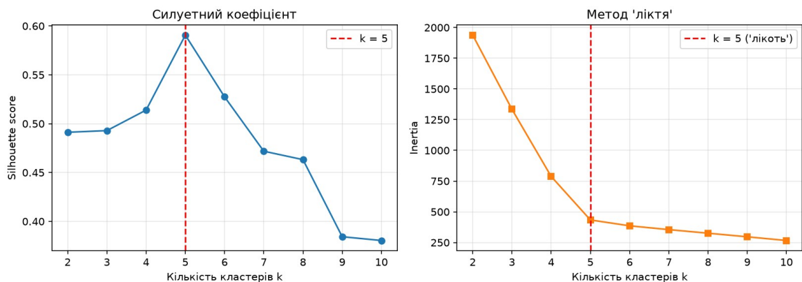
Рисунок 3 — Залежність силуетного коефіцієнта та інерції від кількості кластерів k
