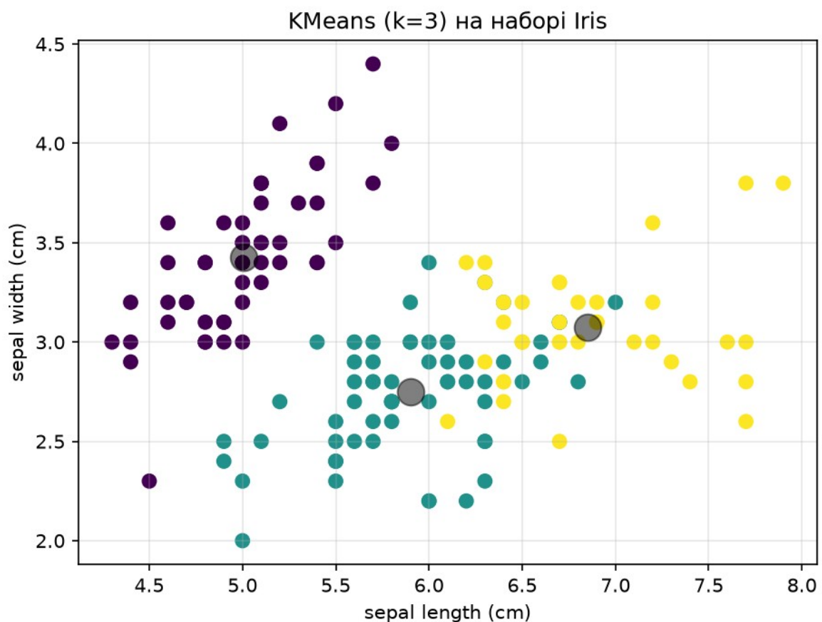
Рисунок 4 — Результат KMeans ( k=3 ) на наборі Iris у площині перших двох ознак
