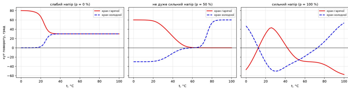
Рисунок 8 — Перерізи поверхонь при трьох рівнях напору: залежність кутів обох кранів від температури води
