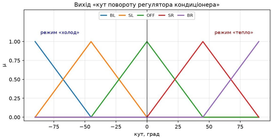
Рисунок 10 — Функції належності виходу «кут повороту регулятора кондиціонера»
