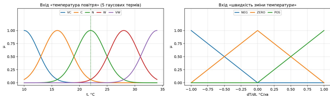
Рисунок 9 — Функції належності входів «температура повітря» і «швидкість зміни температури»
