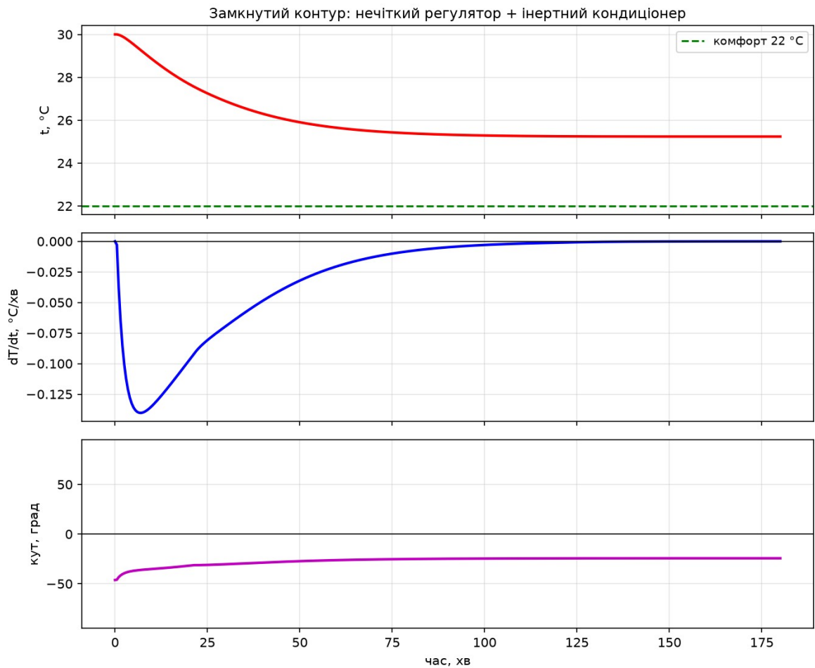
Рисунок 12 — Перевірка в замкнутому контурі: нечіткий регулятор керує інертною моделлю приміщення
