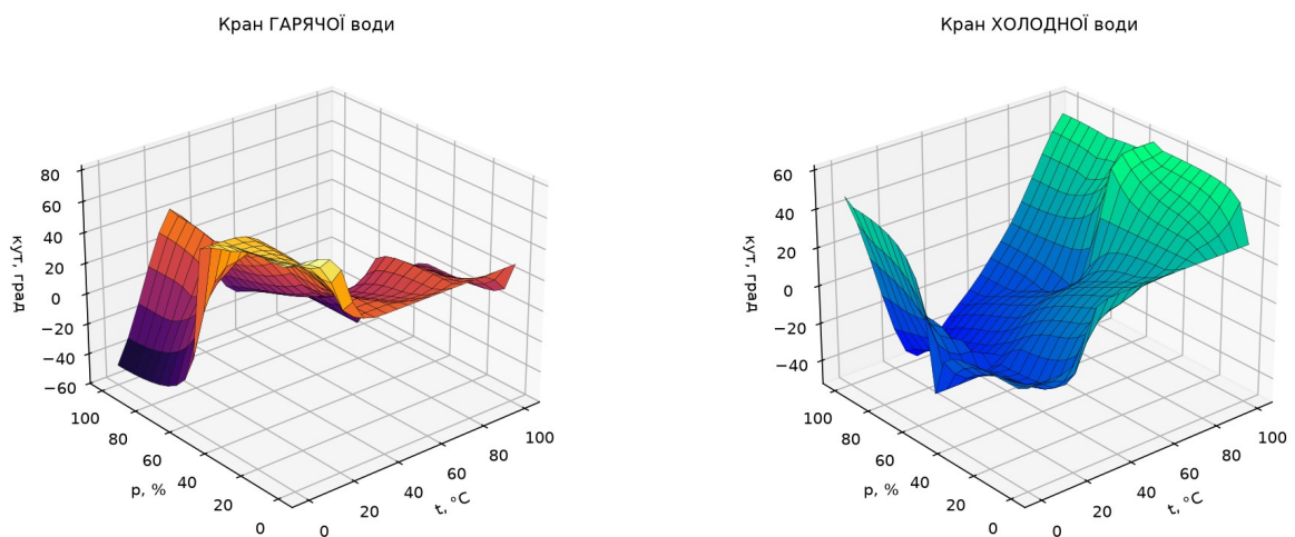
Рисунок 7 — Поверхні «входи-вихід» для обох кранів
