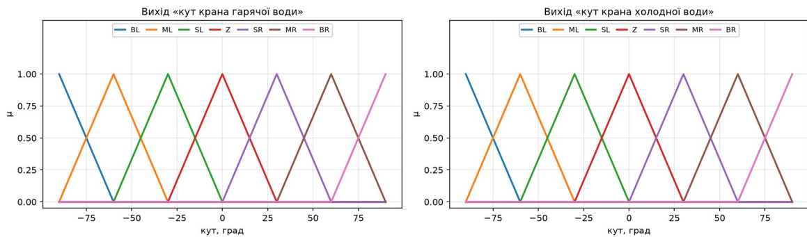
Рисунок 6 — Функції належності вихідних змінних — кутів повороту крана гарячої та крана холодної води
