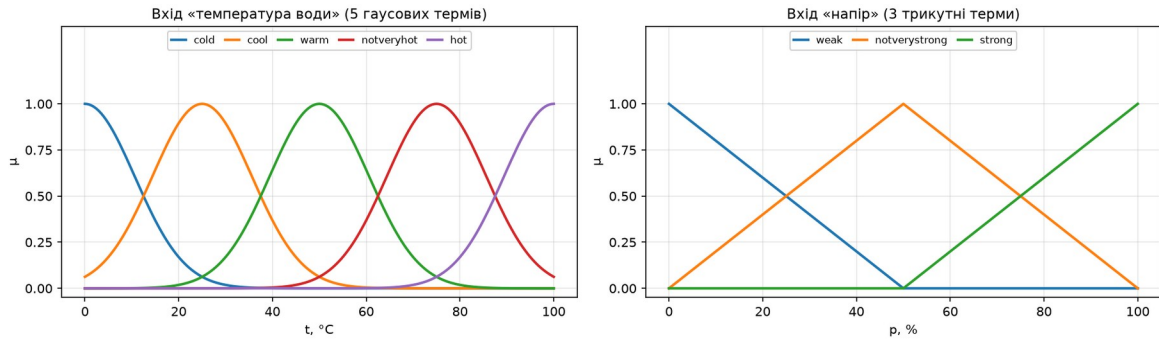
Рисунок 5 — Функції належності вхідних змінних «температура води» і «напір»
