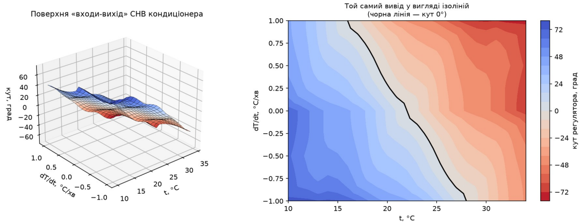
Рисунок 11 — Поверхня «входи-вихід» СНВ кондиціонера та її ізолінії; чорна лінія — межа перемикання між режимами «холод» і «тепло»
