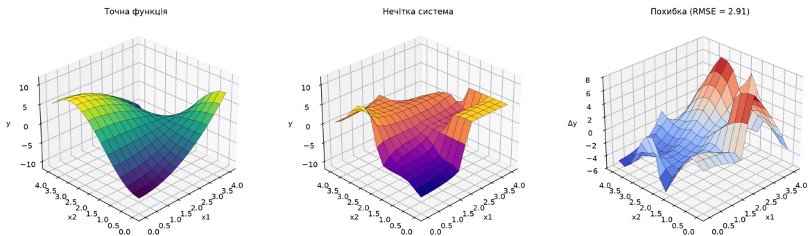
Рисунок 4 — Порівняння: точна функція, нечітка апроксимація та поле похибки
