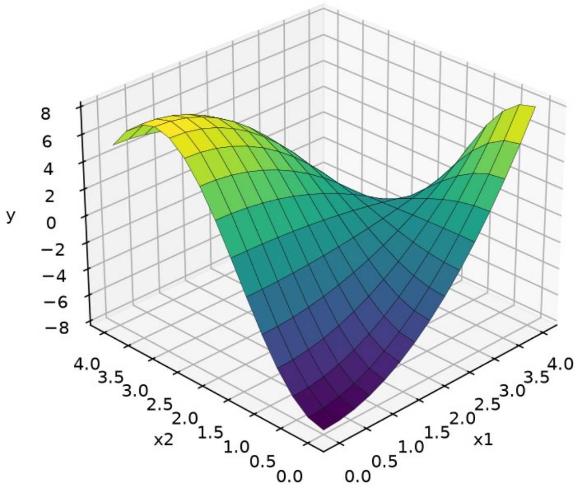
Рисунок 1 — Точна поверхня y = (x_1^2 - 8) \cdot \cos(x_2) на області x_1, x_2 \in [0, 4] (аналог команди surf)
