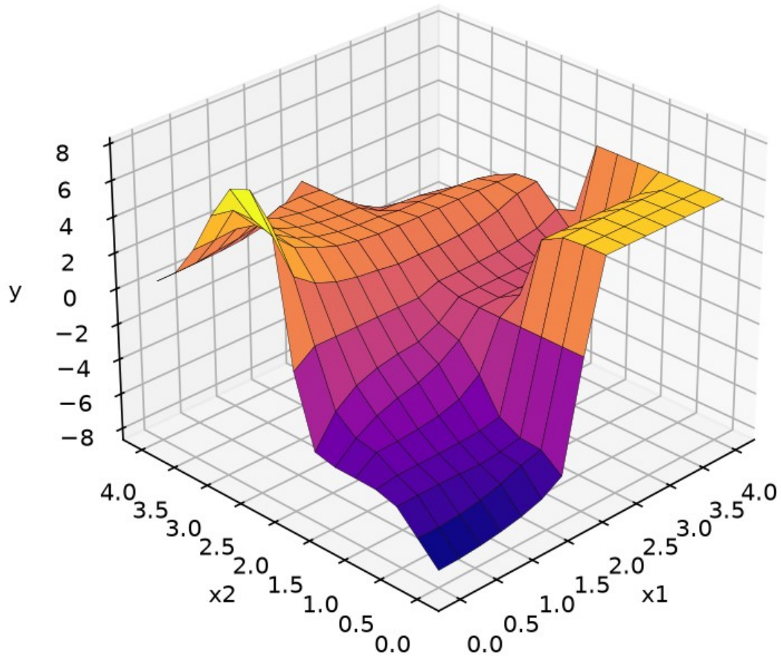
Рисунок 3 — Поверхня «входи-вихід» синтезованої системи нечіткого виводу (аналог вікна View surface...)
