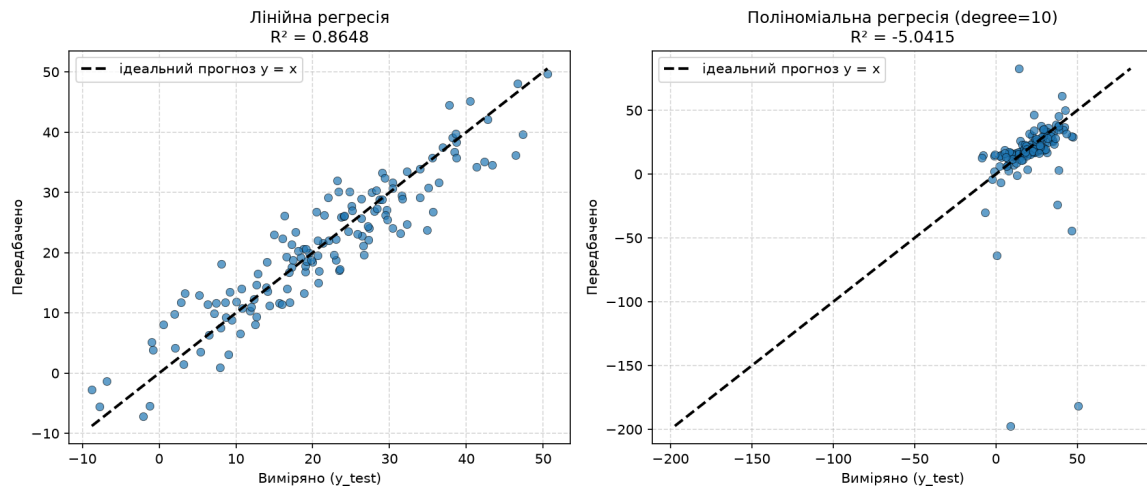
Рисунок 5 — багатовимірна регресія: лінійна (ліворуч) та поліноміальна degree=10 (праворуч)
