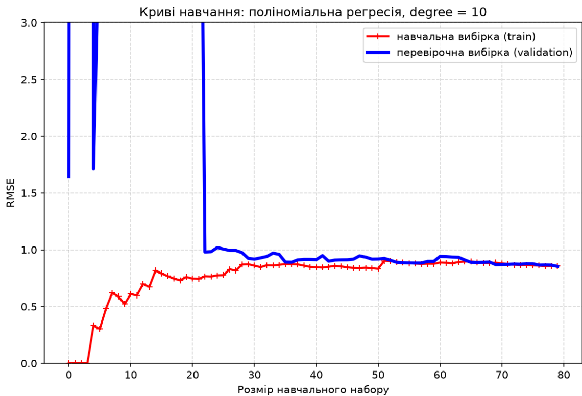
Рисунок 10 — криві навчання поліноміальної моделі degree = 10
