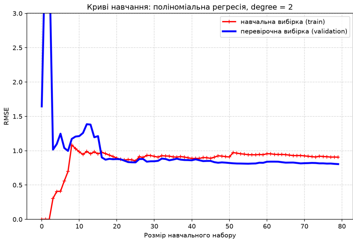
Рисунок 9 — криві навчання поліноміальної моделі degree = 2
