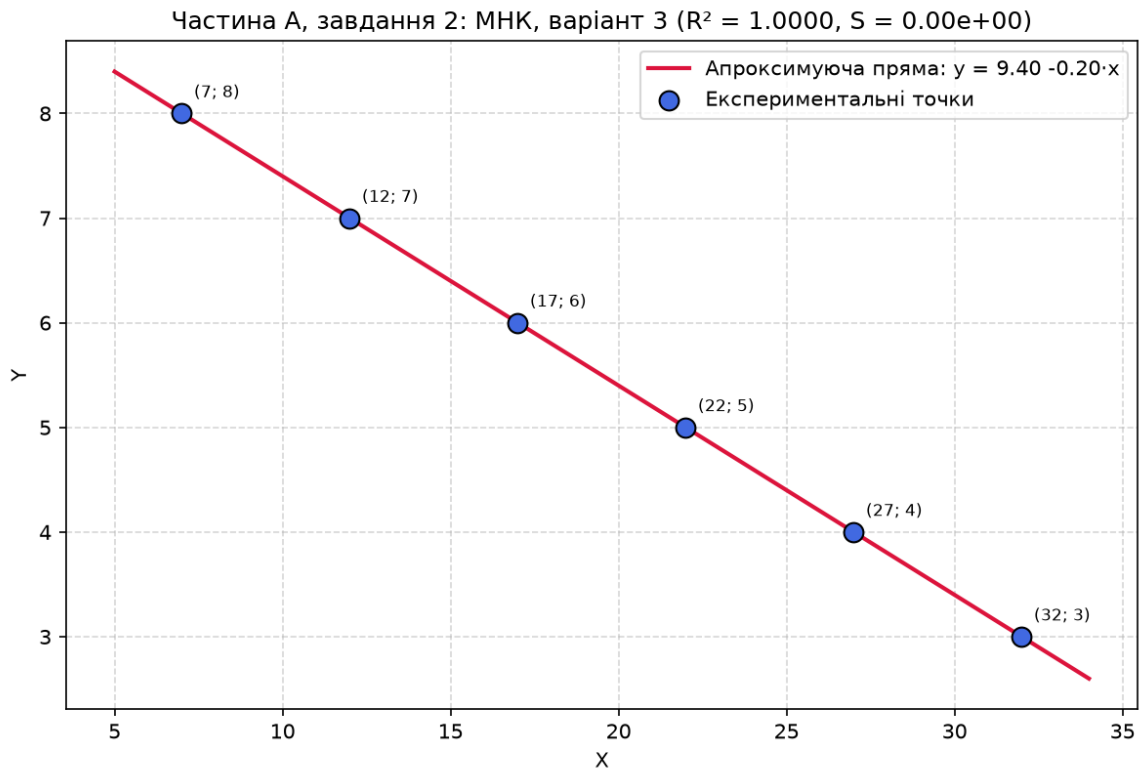
Рисунок 1 — МНК для варіанта 3: експериментальні точки та апроксимуюча пряма
