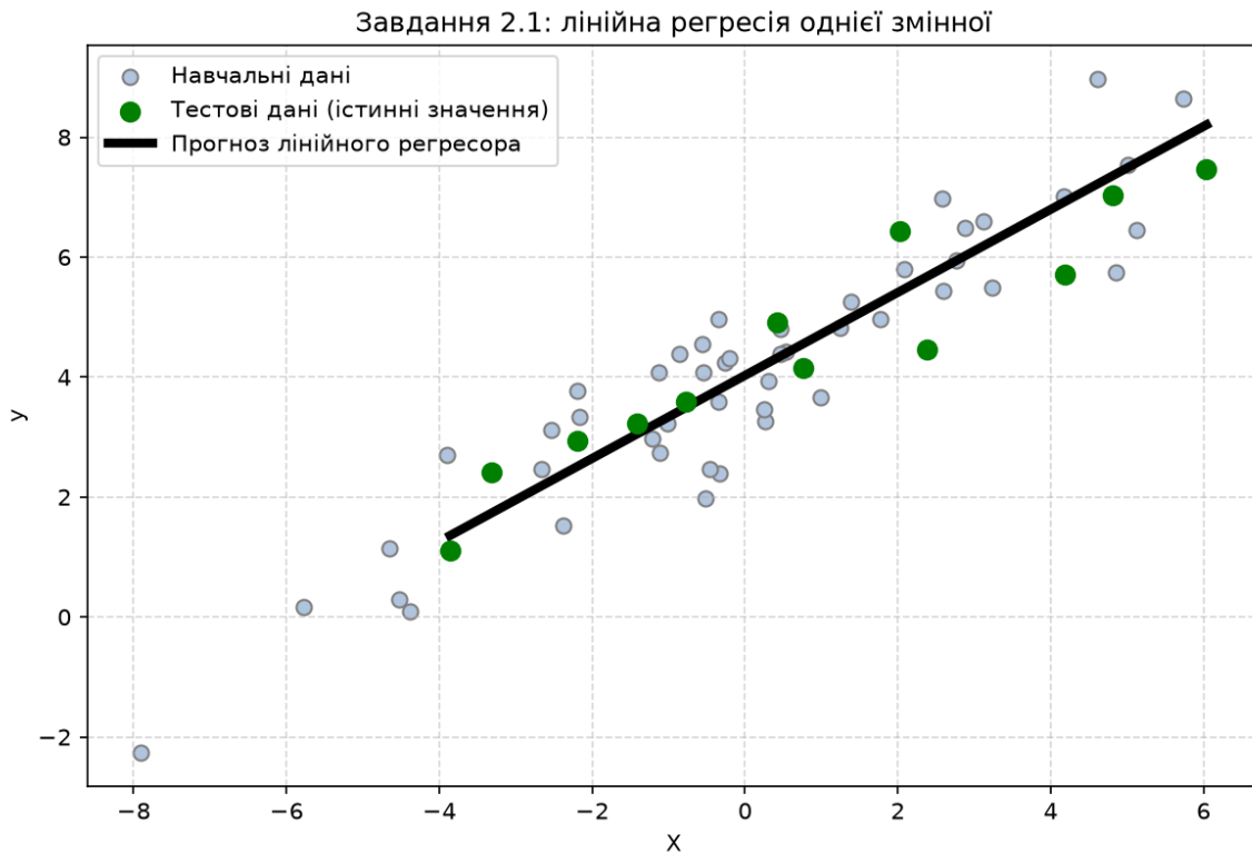
Рисунок 3 — лінійна регресія однієї змінної (завдання 2.1)
