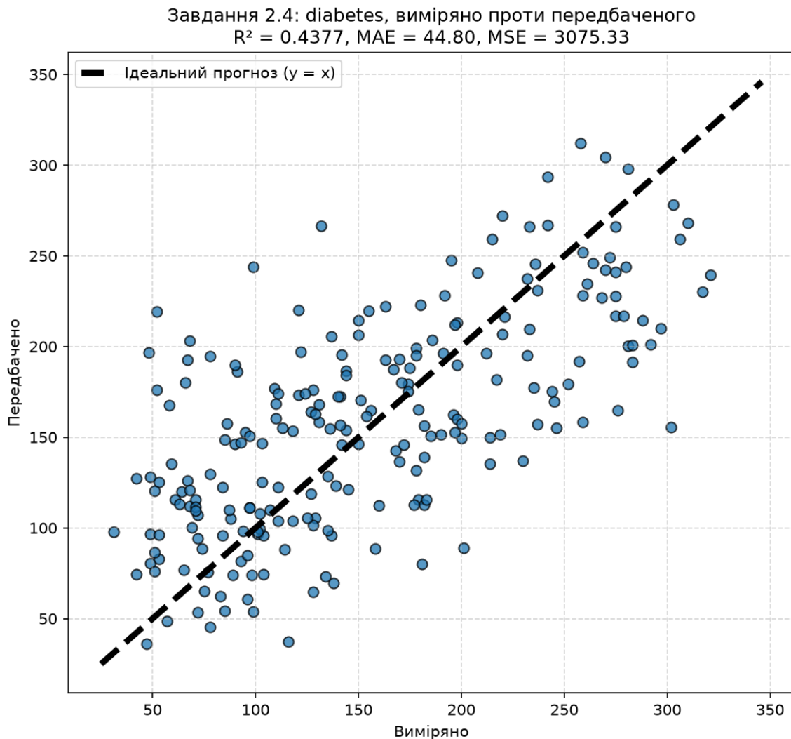
Рисунок 6 — diabetes: виміряні проти передбачених значень із лінією y = x
