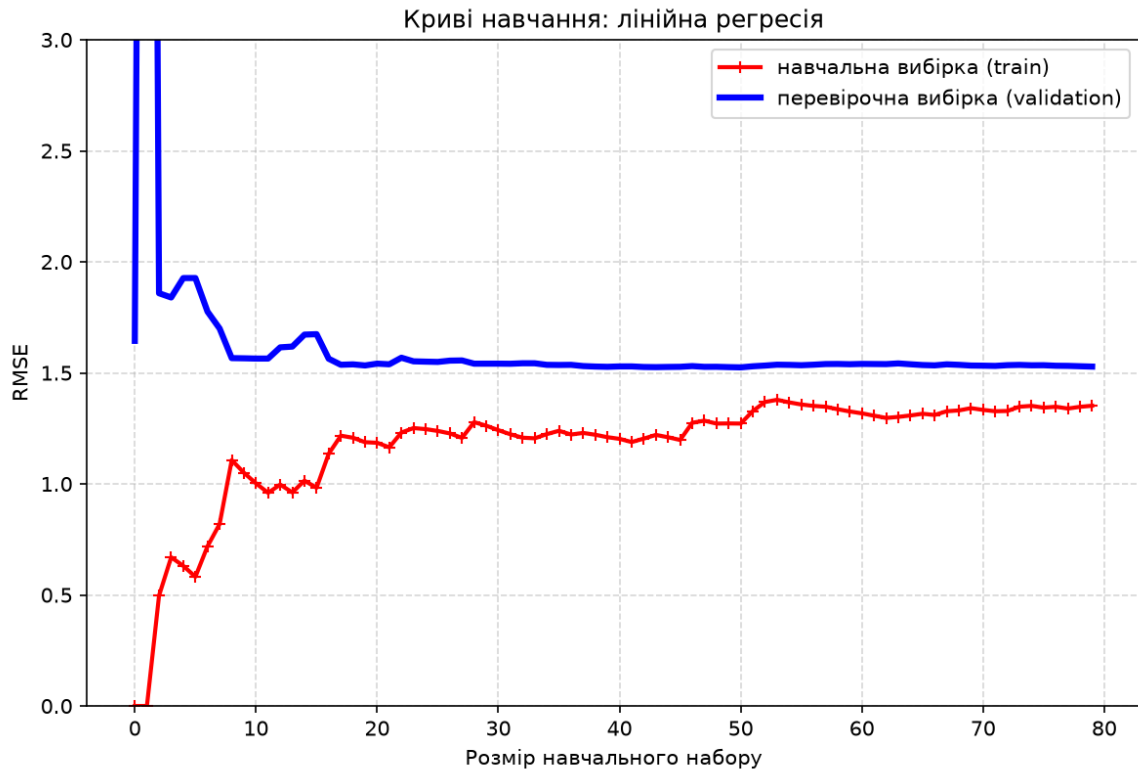
Рисунок 8 — криві навчання лінійної моделі
