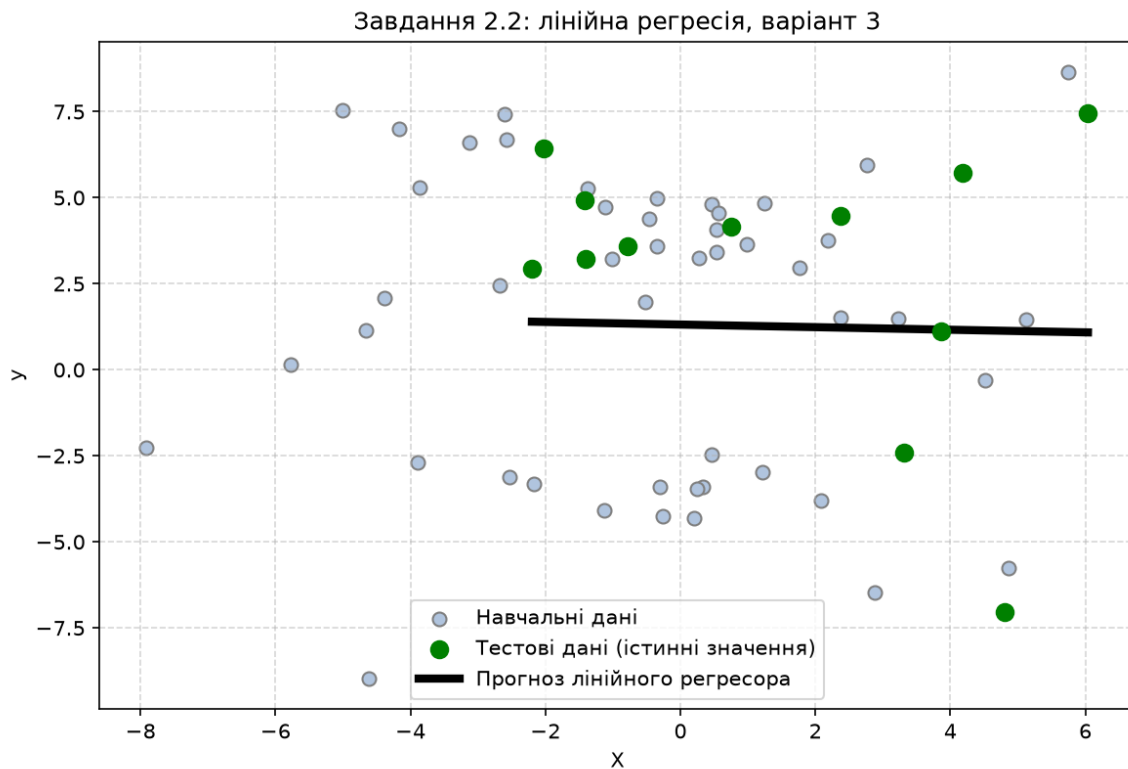
Рисунок 4 — лінійна регресія на даних варіанта 3
