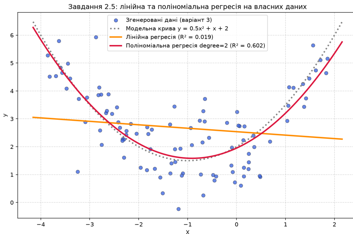
Рисунок 7 — власні дані варіанта 3: лінійна та поліноміальна регресія
