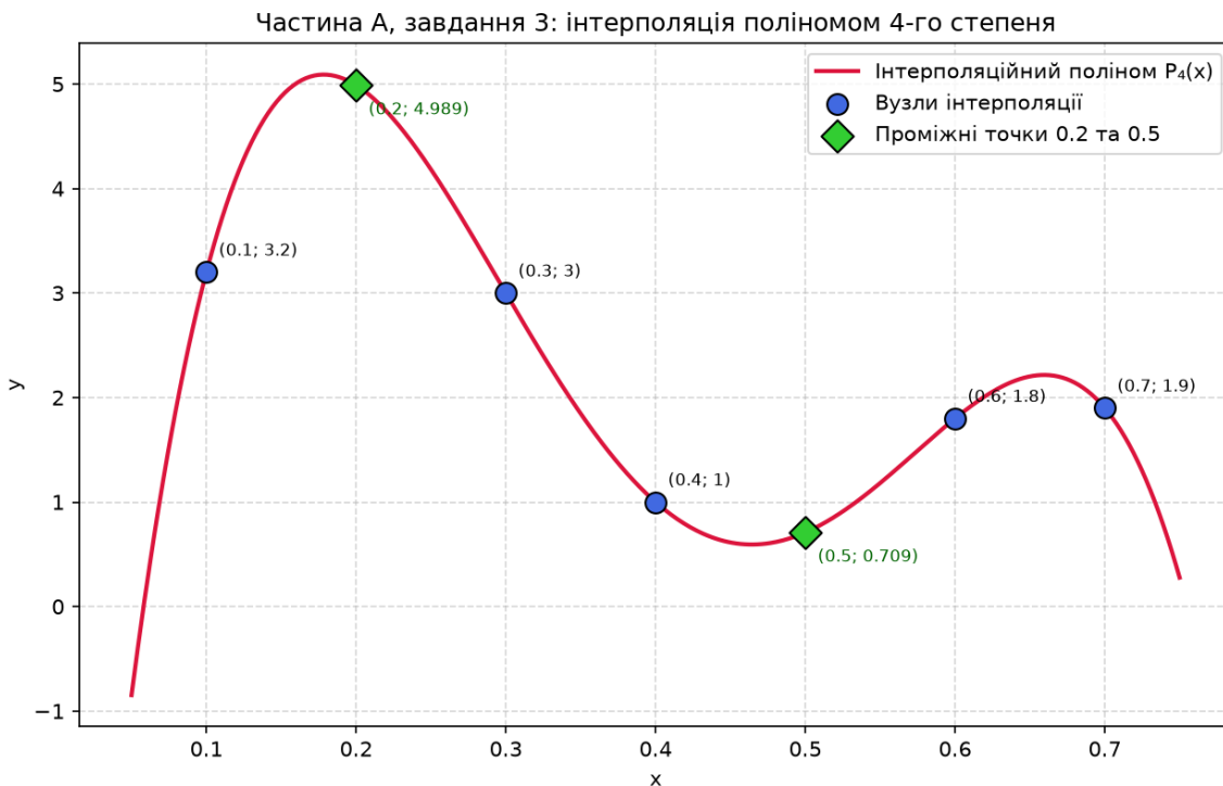
Рисунок 2 — інтерполяційний поліном 4-го степеня та значення у точках 0.2 і 0.5
