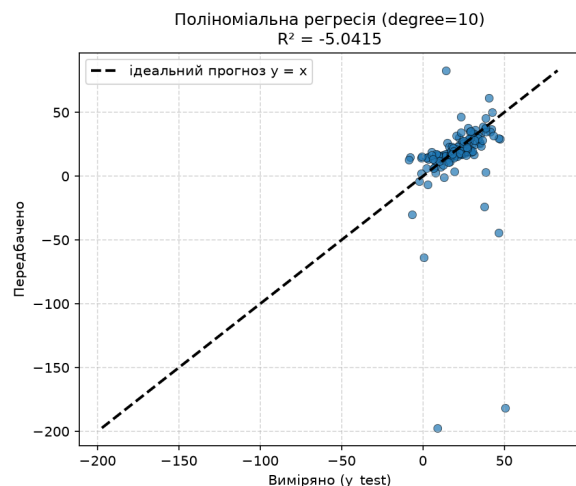
Рисунок 5 — багатовимірна регресія: лінійна (ліворуч) та поліноміальна degree=10 (праворуч)
