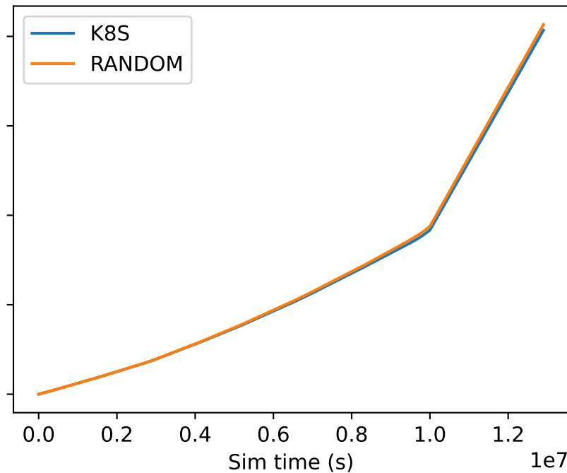
Scenario: HIGH
