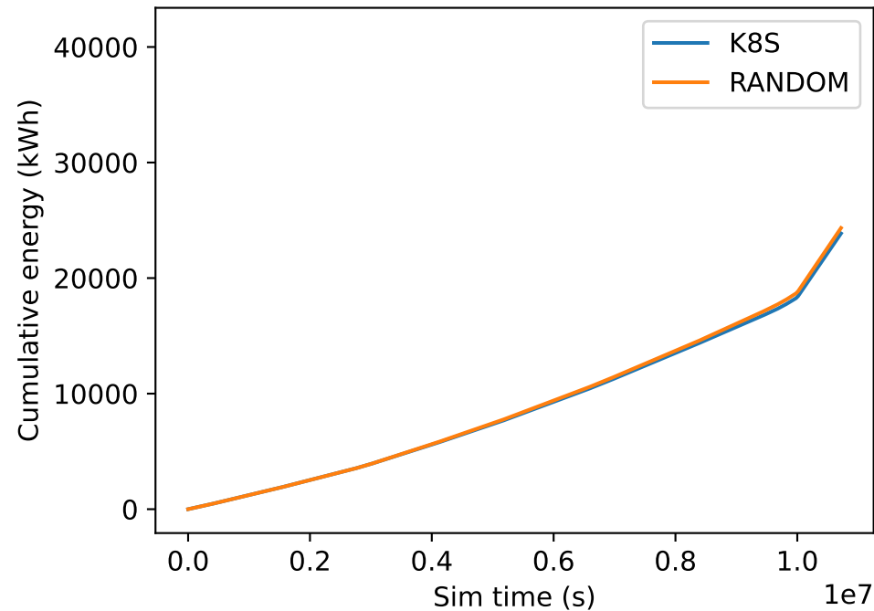
Scenario: LOW
