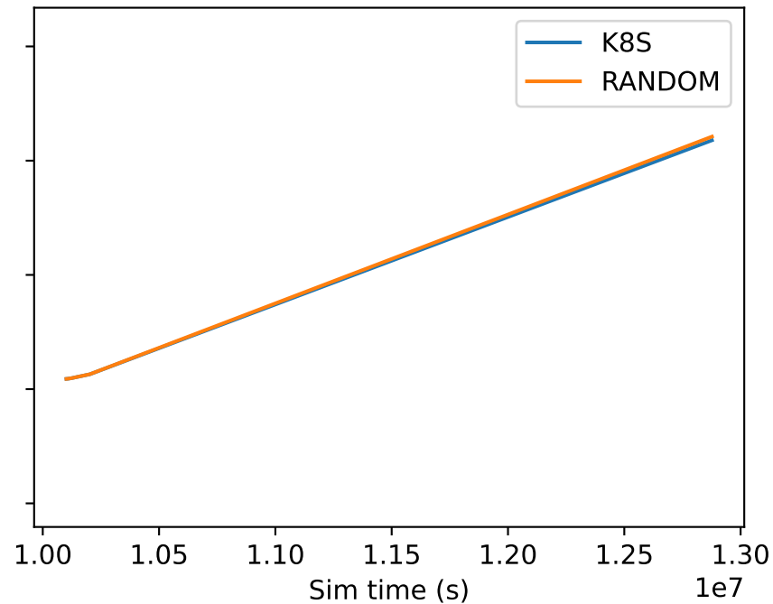
Scenario: BURST
