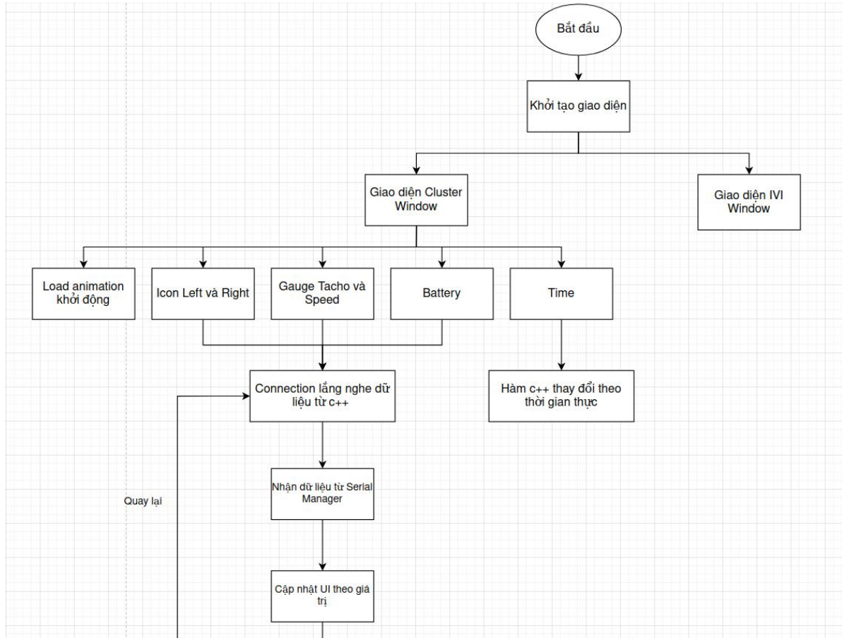
Hình 3.3-2. Lưu đồ thuật toán giao diện Cluster
