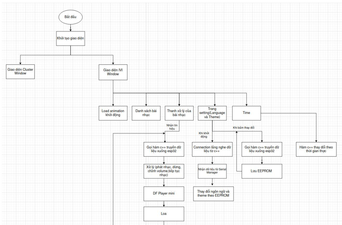
Hình 3.3-3. Lưu đồ thuật toán giao diện IVI
