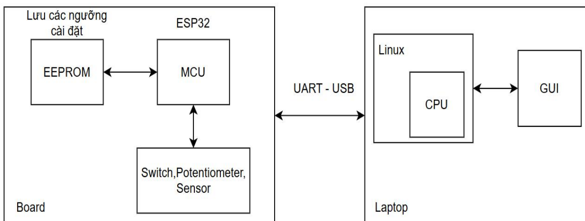
Hình 2.2-1. Mô hình hệ thống
