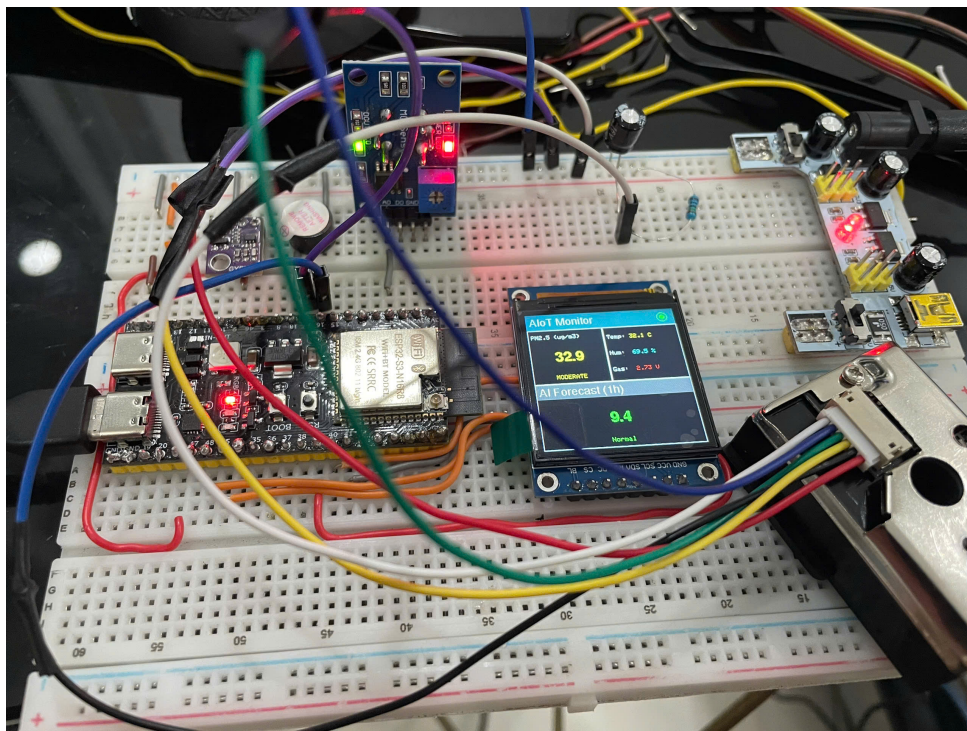
Hình 6: Hệ thống phần cứng hoàn chỉnh: ESP32-S3 tích hợp ba cảm biến môi trường, màn hình IPS ST7789, còi buzzer và LED cảnh báo
